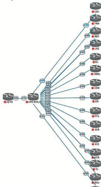
Gráfico N° 5 Diagrama de la Red VPN-MPLS de la AETN
