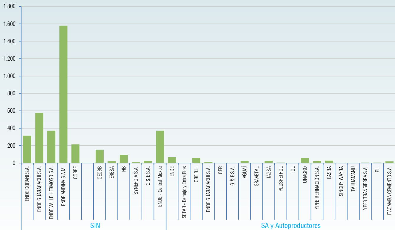
Gráfico I-3 Potencia Instalada por empresa (MW) Gestión 2024 - SIN y SA
