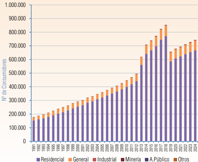
Gráfico V-13 Evolución número de Consumidores Periodo (1991-2024) - DELAPAZ
