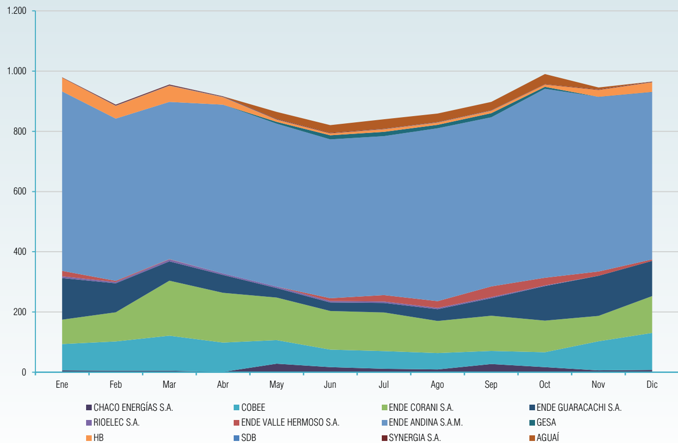
Gráfico I-8 Evolución mensual de la Generación Bruta en el SIN (GWh) Gestión 2024
