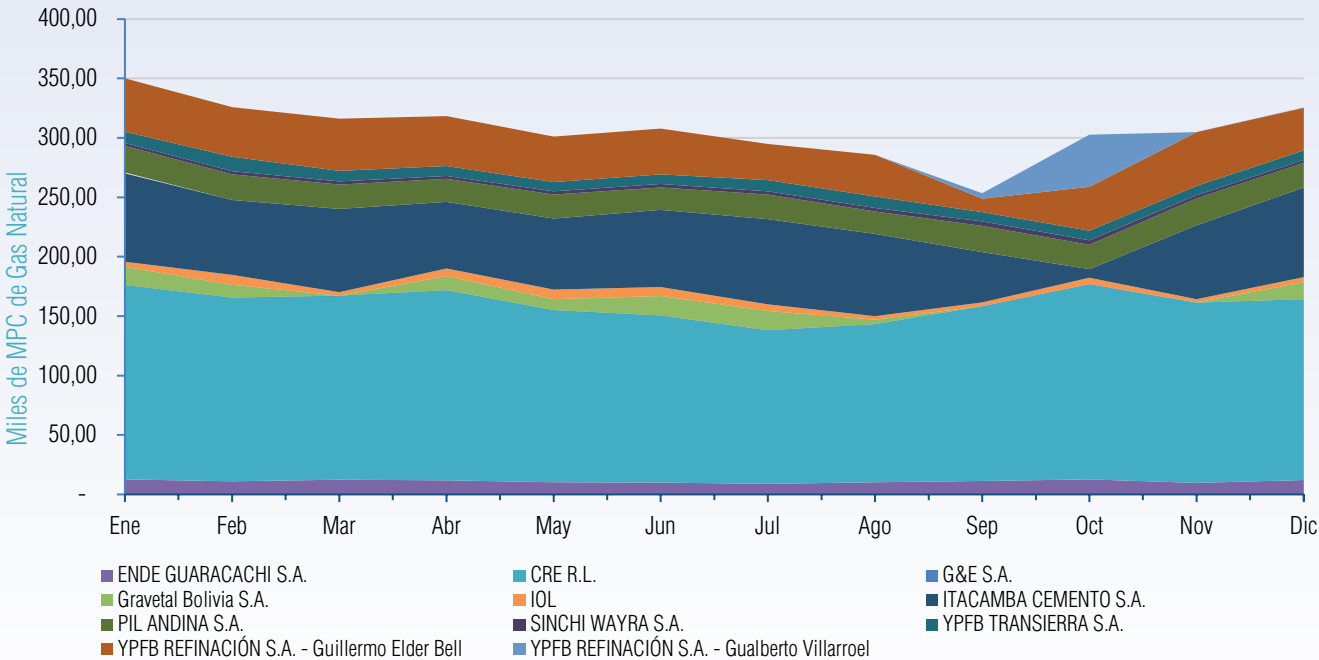
Gráfico VI-13 Evolución mensual consumo de Gas Natural (MMPC) Gestión 2024 - Sistemas Aislados
