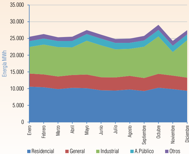
Gráfico V-58 Evolución mensual de ventas de Energía Gestión 2024 - CESSA
