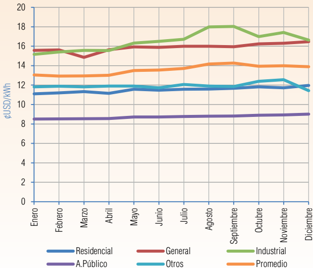
Gráfico V-132 Evolución mensual de la Tarifa Promedio Gestión 2024 - ENDE (Uyuni)
