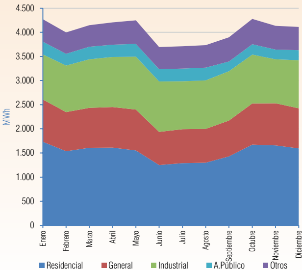
Gráfico V - 307 Evolución mensual de las ventas de Energía Gestión 2024 -CRE R.L. (San Ignacio de Velasco)
