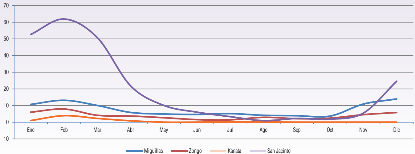
Gráfico IV-13 Aportes a los embalses (hm³) - Miguillas, Zongo, Kanata y San Jacinto Gestión 2024
