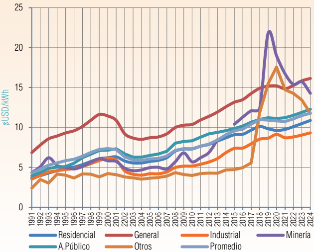
Gráfico V-11 Evolución de la Tarifa Promedio Periodo (1991 - 2024) - DELAPAZ
