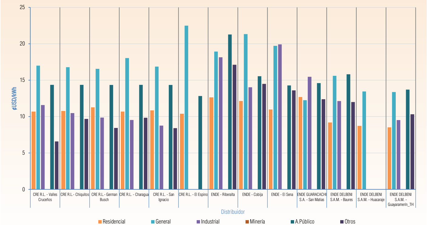
Gráfico V - 277 Tarifa Promedio a consumidor final Gestión 2024 - SA
