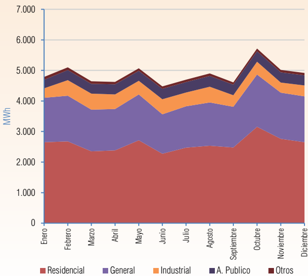
Gráfico V - 319 Evolución mensual de las ventas de Energía Gestión 2024 - ENDE - RIBERALTA
