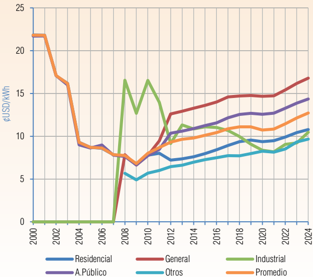
Gráfico V - 290 Evolución de la Tarifa Promedio Periodo (2000 - 2024) - CRE R.L.(Chiquitos)
