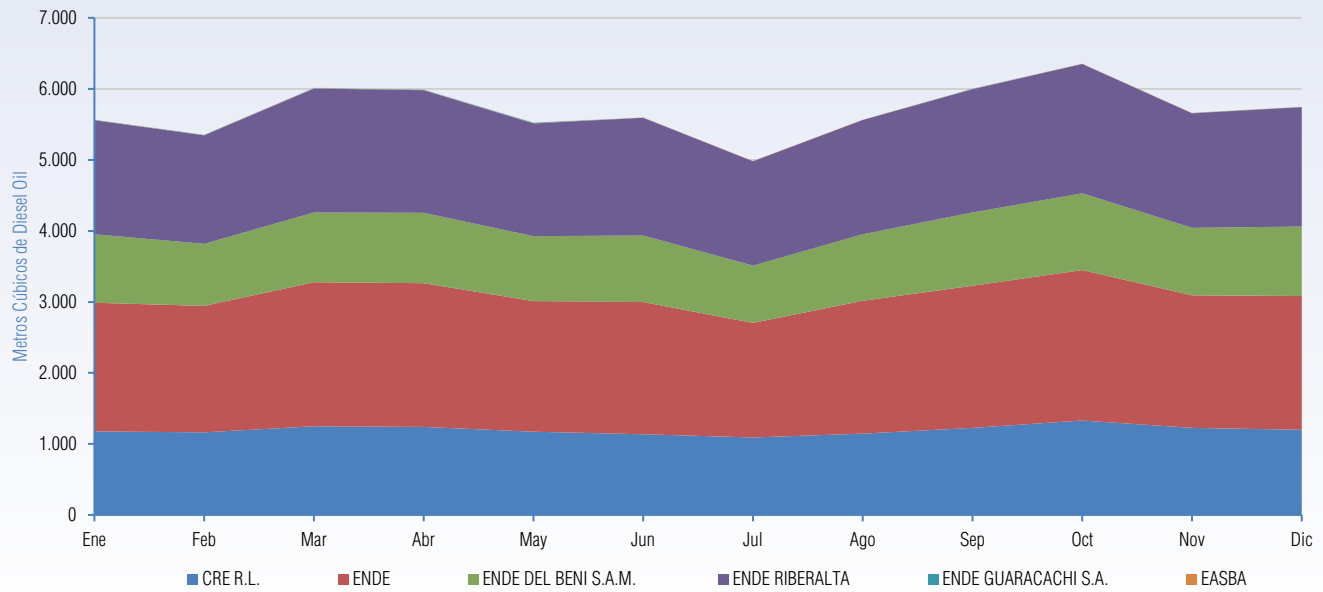
Gráfico VI-14 Evolución mensual consumo de Diesel Oil (m³) Gestión 2024 - Sistemas Aislados
