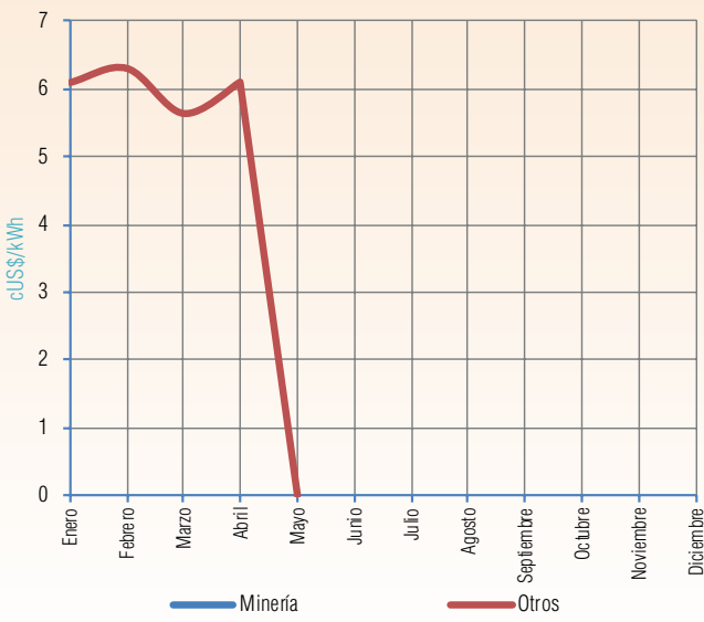
Gráfico V-258 Evolución Mensual de la Tarifa Promedio Gestión 2021 - SEPSA (Sistema Sur)
