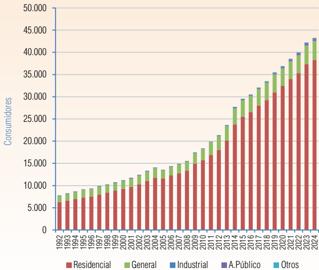
Gráfico V-85 Evolución del número de Consumidores Periodo (1992 - 2024) - ENDE DELBENI S.A.M. (Trinidad)
