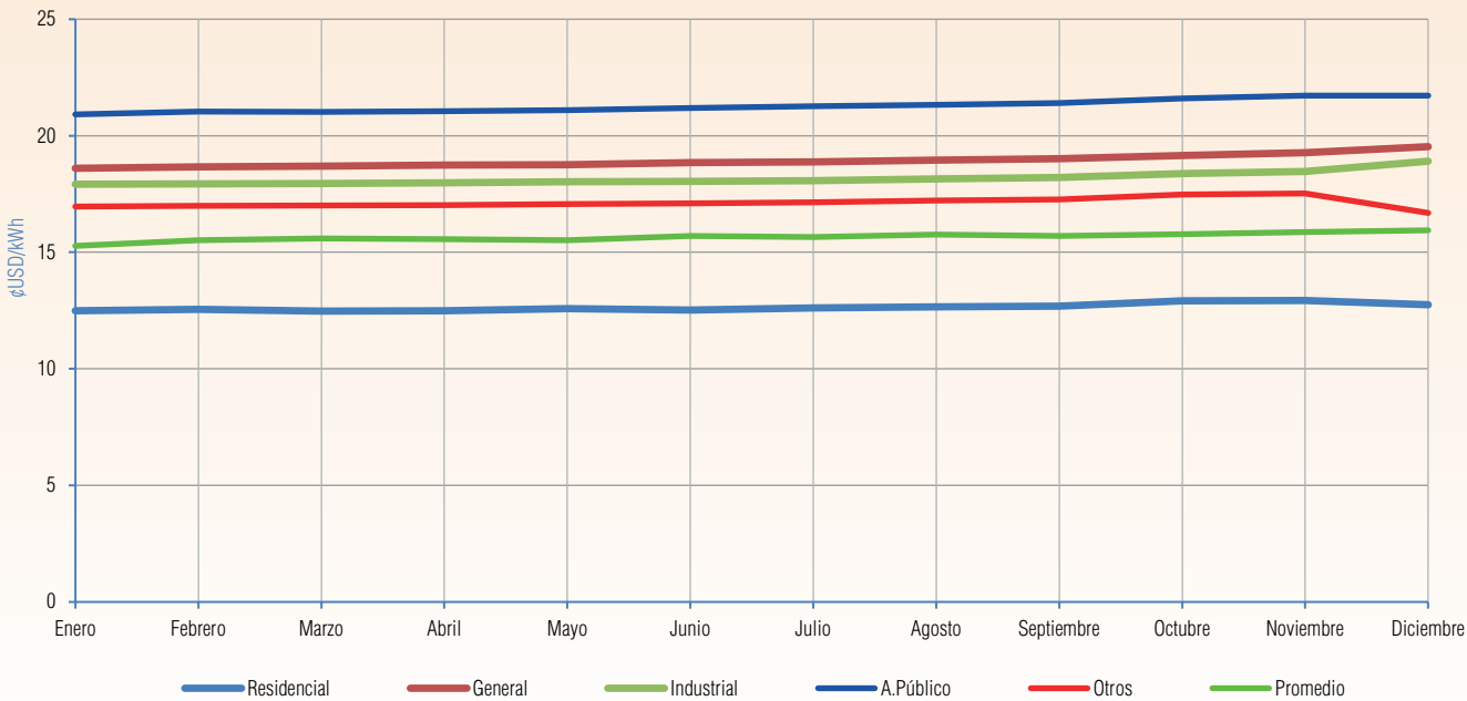
Gráfico V - 502 Evolución mensual de la Tarifa Promedio Gestión 2024 - ENDE (Riberalta)
