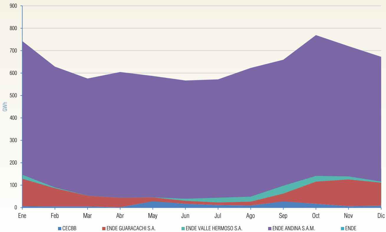
Gráfico II-12 Generación Termoeléctrica de las empresas (GWh) Gestión 2024 - SIN
