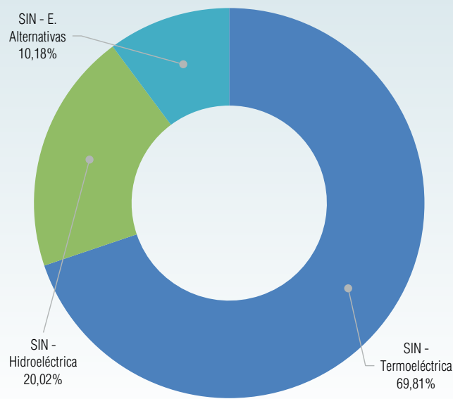
Gráfico I-1 Potencia Instalada por tipo de tecnología (%) Gestión 2024 - SIN
