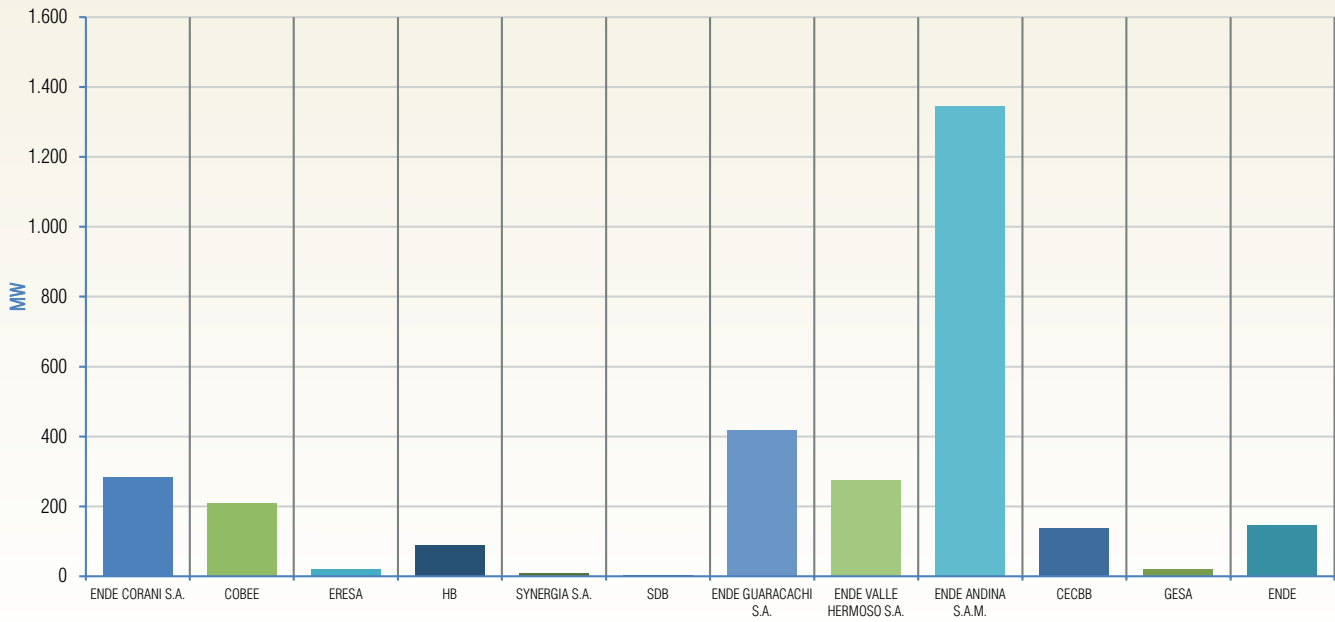
Gráfico II-4 Participación de las empresas de generación en el parque generador del SIN (MW) Gestión 2024
