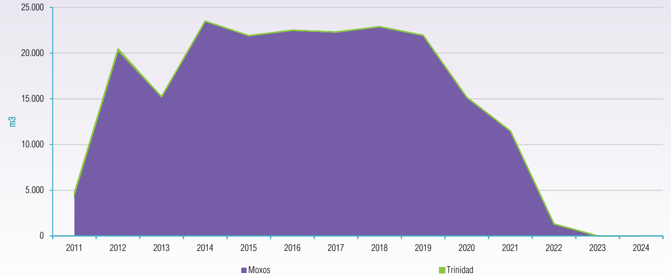
Gráfico IV - 8 Evolución anual del consumo de Diesel Oil en las centrales: Moxos y Trinidad Período 2011 - 2024
