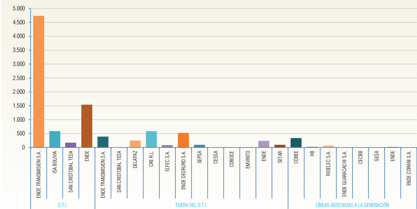
Gráfico II-6 Longitud de Línea de Transmisión (Km) Gestión 2024
