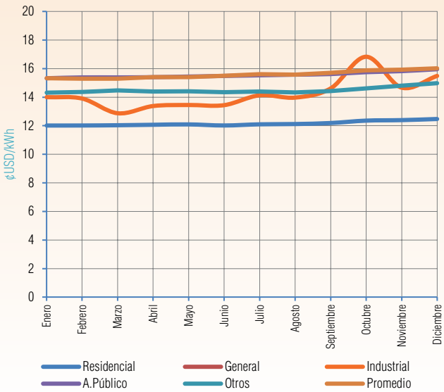
Gráfico V - 327 Evolución Mensual de la Tarifa Promedio Gestión 2024 - ENDE (Cobija)
