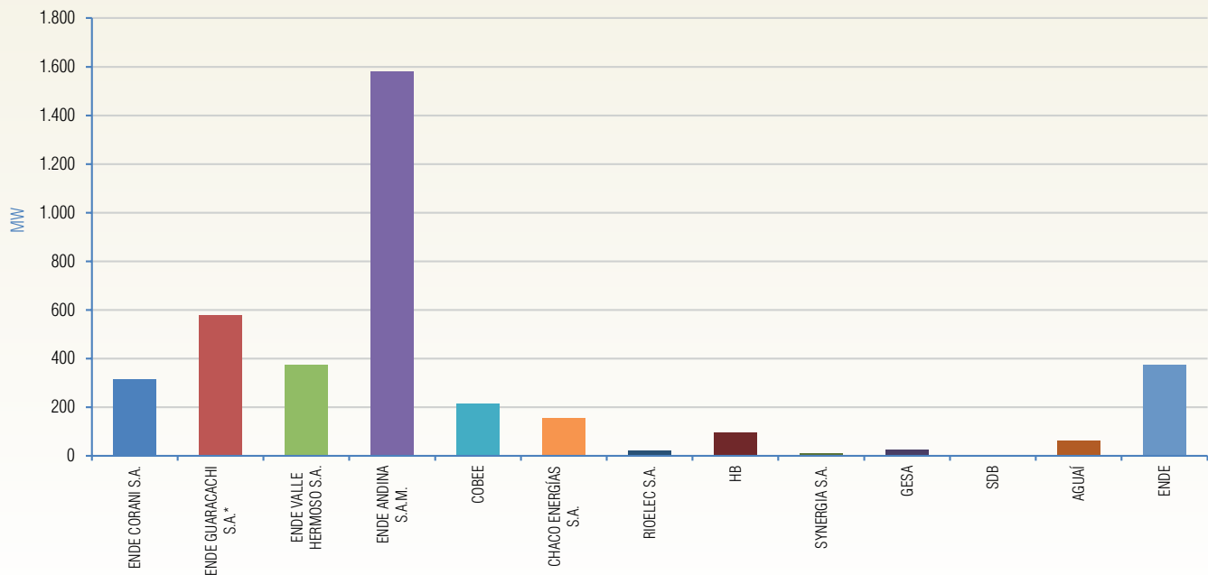
Gráfico II-2 Participación de las empresas del SIN Potencia Instalada (MW) Gestión 2024 - SIN
