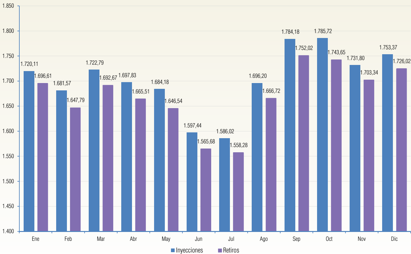
Gráfico II-19 Potencia Máxima (MW) Gestión 2024 - MEM
