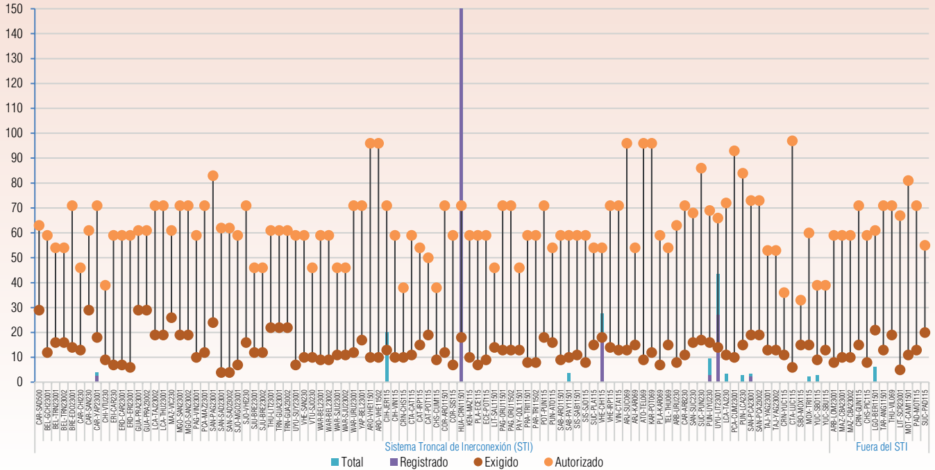
Gráfico VII-2 Duración Media de Desconexiones (minutos) Periodo (Nov/2023-Oct/2024) - Calidad de Transmisión
