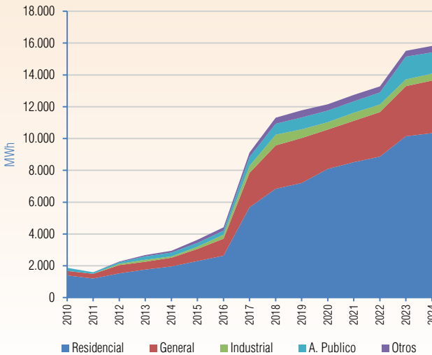
Gráfico V-93 Evolución de ventas de Energía Periodo (2010 - 2024) - ENDE DELBENI S.A.M. (San Ignacio de Moxos)
