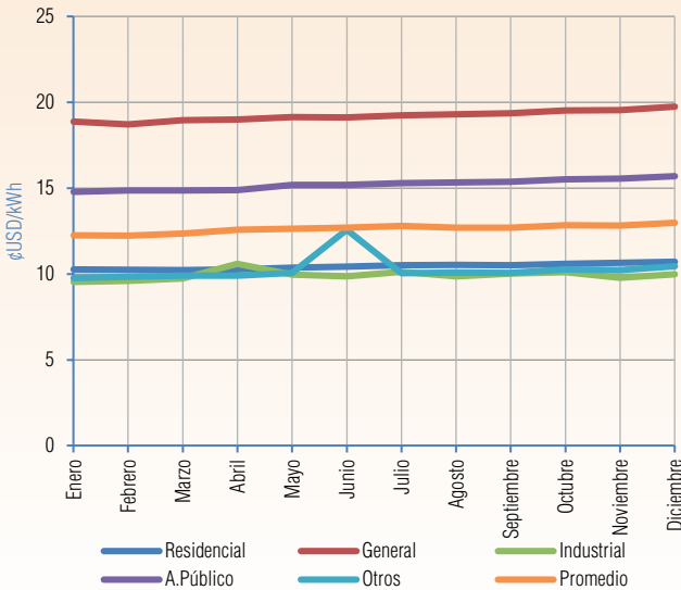
Gráfico V-138 Evolución mensual de la Tarifa Promedio Gestión 2024 - SETAR (Tarifa)
