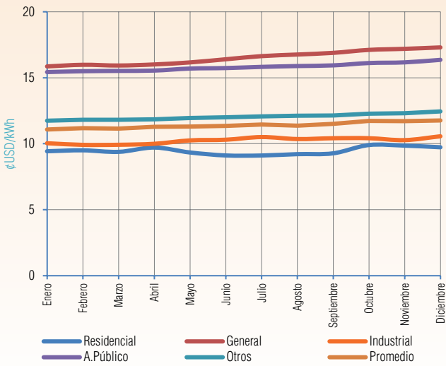
Gráfico V-102 Evolución Mensual de la Tarifa Promedio Gestión 2024 - ENDE DELBENI S.A.M. (San Borja)
