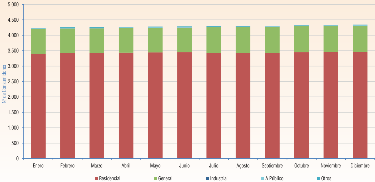
Gráfico V - 506 Evolución mensual del número de Consumidores Gestión 2024 - ENDE GUARACACHI S.A. (San Matías)
