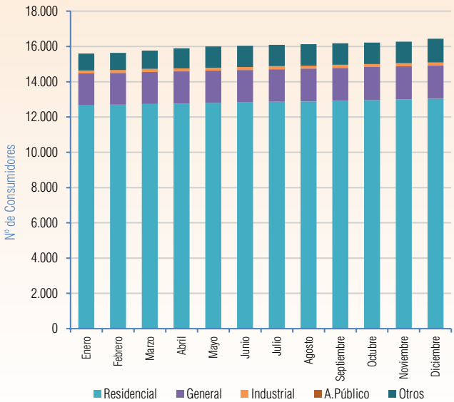
Gráfico V - 311 Evolución mensual de número de Consumidores Gestión 2024 - CRE R.L. (San Ignacio de Velasco)
