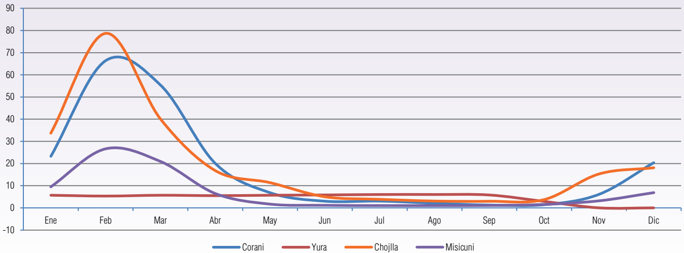
Gráfico IV - 12 Aportes a los embalses (hm³) - Corani, Yura, Chojlla y Misicuni Gestión 2024
