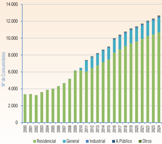
Gráfico V - 298 Evolución número de Consumidores Periodo (2000 - 2024) - CRE R.L. (G. Busch)
