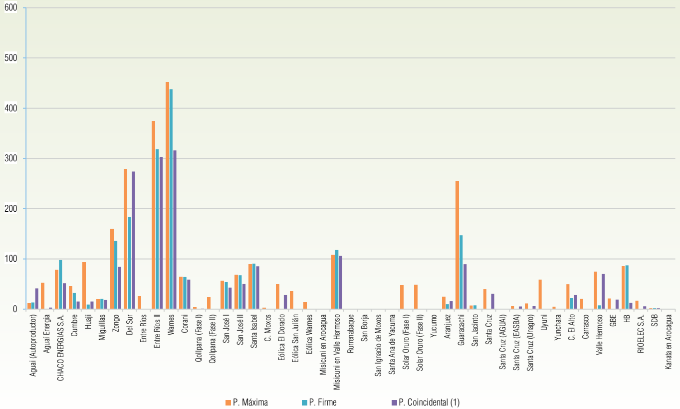
Gráfico III - 3 Potencias inyectadas por central (MW) Gestión 2024 - MEM
