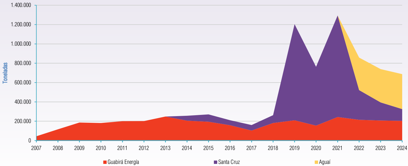
Gráfico IV - 10 Evolución anual del consumo de Biomasa en las centrales: Guabirá y Santa Cruz Período 2007-2024
