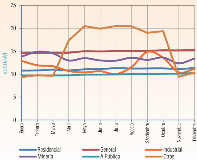
Gráfico V-24 Evolución mensual de la Tarifa Promedio Gestión 2024 - DELAPAZ (Larecaja)
