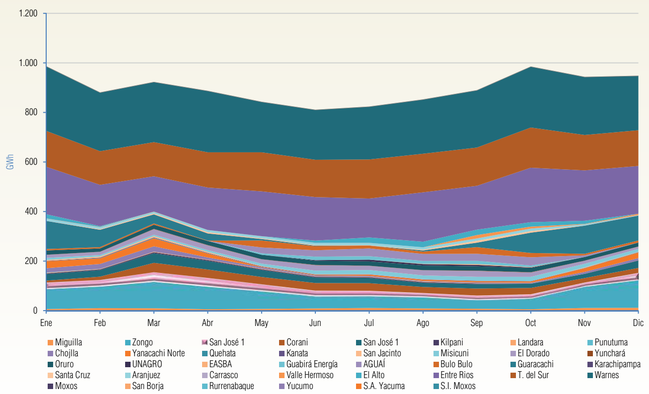
Gráfico II-9 Evolución mensual Generación Bruta de Centrales (GWh) Gestión 2024 - SIN
