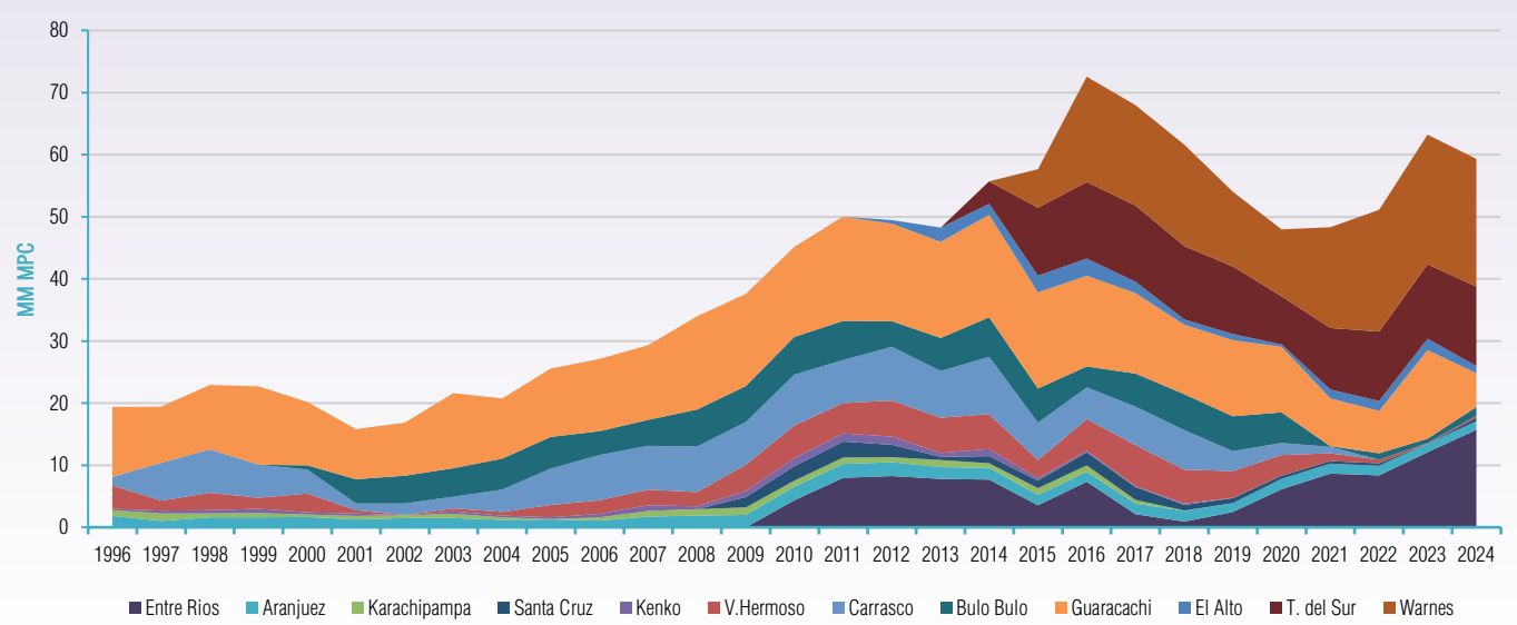
Gráfico IV - 6 Evolución anual del consumo de Gas Natural Período 1996-2024
