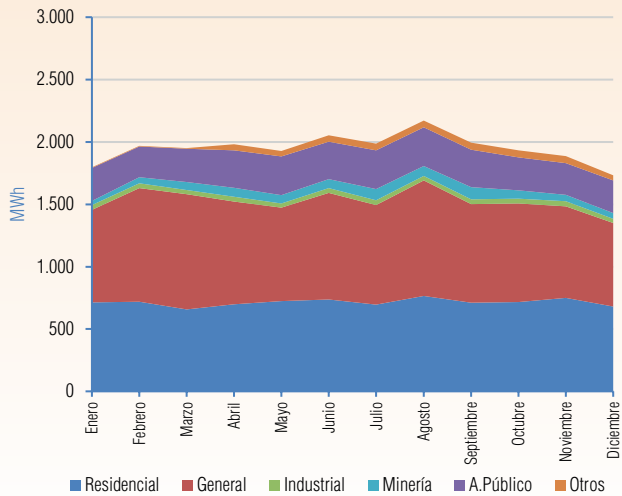
Gráfico V-16 Evolución mensual de ventas de Energía Gestión 2024 - DELAPAZ (Aroma)
