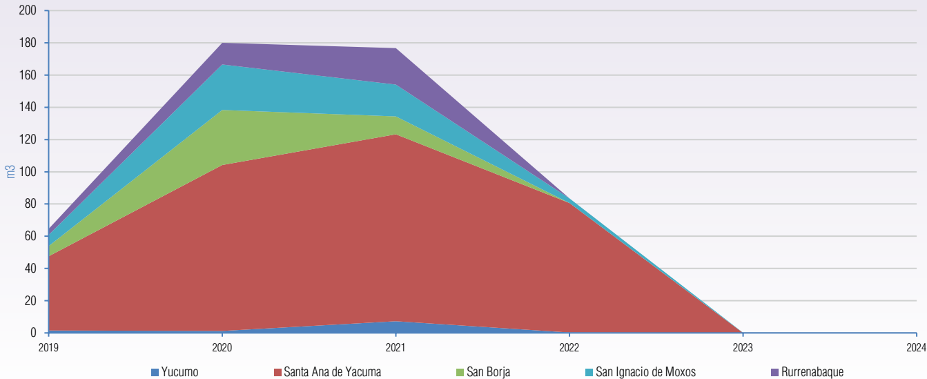
Gráfico IV - 9 Evolución anual del consumo de Diesel Oil en las centrales: Yucumo, Santa Ana de Yacuma, San Borja, San Ignacio de Moxos y Rurrenabaque Período 2019 - 2024
