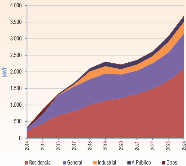
Gráfico V - 330 Evolución de las ventas de Energía Periodo (2014 - 2024) - ENDE (El Sena)
