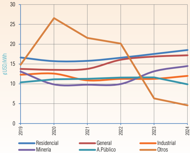
Gráfico V-17 Evolución de la Tarifa Promedio Periodo (2019 - 2024) - DELAPAZ (Aroma)
