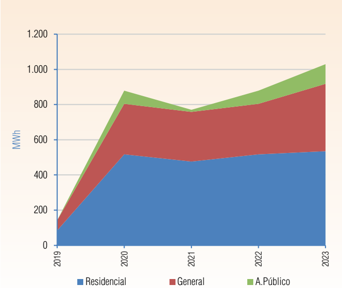
Gráfico V - 366 Evolución de las ventas de Energía Periodo (2019 - 2023) - ENDE (Puerto Gonzalo Moreno)
