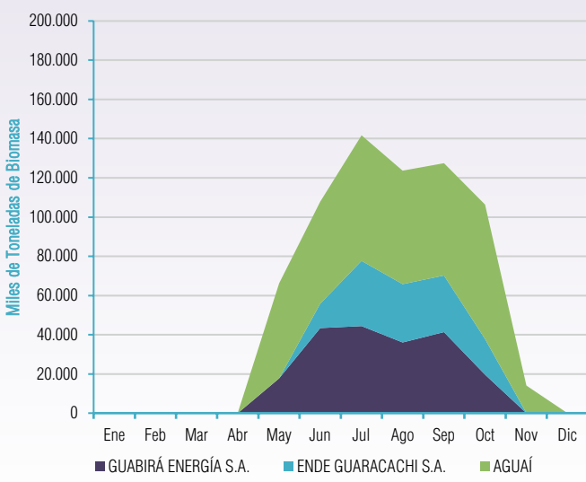
Gráfico IV-5 Evolución mensual del consumo de Biomasa Gestión 2024
