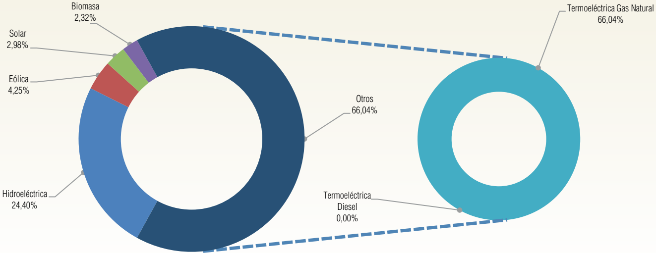
Gráfico II-7 Generación Bruta - SIN Participación por tipo de tecnología - Gestión 2024
