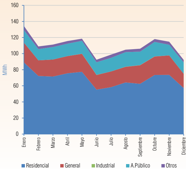
Gráfico V - 343 Evolución de las ventas de Energía Gestión 2024 - ENDE DELBENI S.A.M. (Baures)
