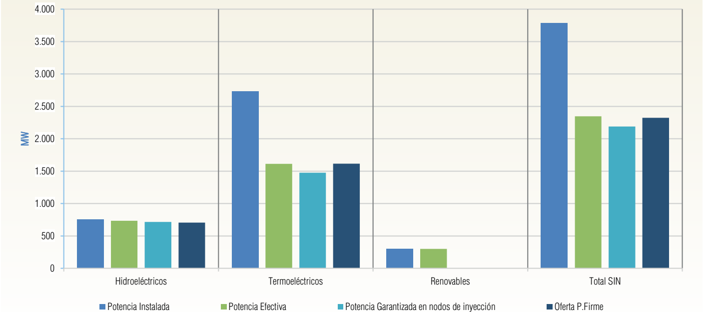
Gráfico II-3 Parque generador declarado disponible en el SIN (MW) Gestión 2024 - SIN
