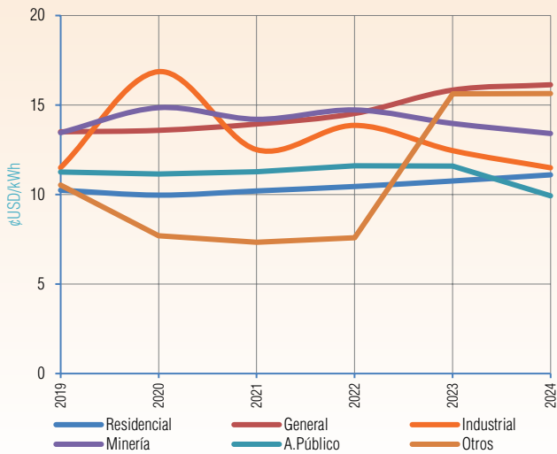
Gráfico V-23 Evolución de la Tarifa Promedio Periodo (2019 - 2024) - DELAPAZ (Larecaja)
