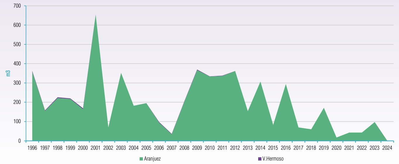
Gráfico IV - 7 Evolución anual del consumo de Diesel Oil en las centrales: Aranjuez y Valle Hermoso Período 1996 - 2024
