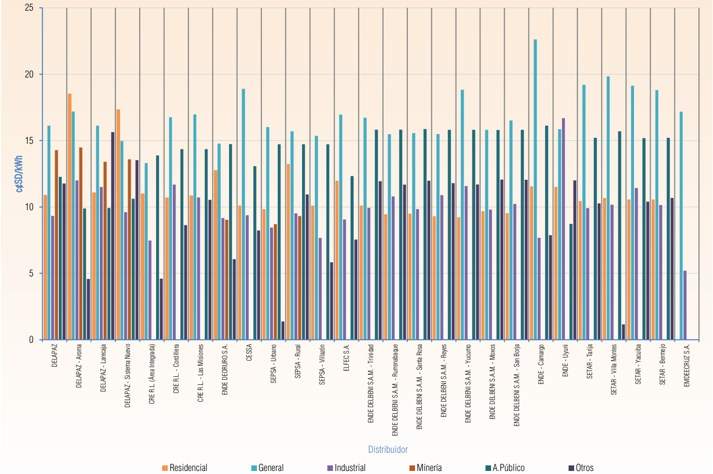
Gráfico V-6 Tarifa Promedio a consumidor final Gestión 2024 - SIN - [¢USD/kWh] (sin IVA)
