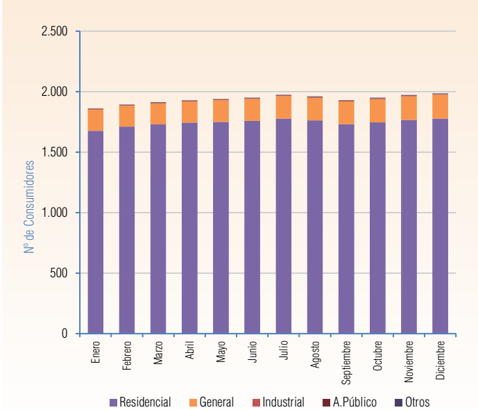
Gráfico V - 335 Evolución mensual del número de Consumidores Gestión 2024 - ENDE (El Sena)
