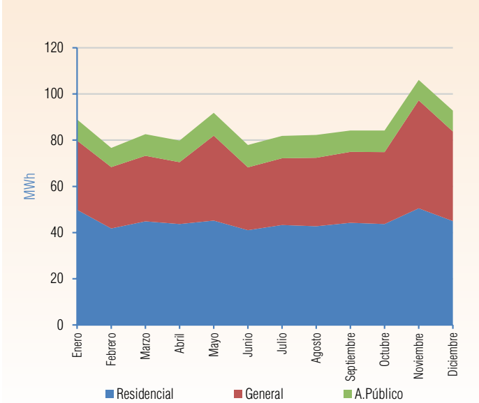
Gráfico V - 367 Evolución mensual de ventas de Energía Gestión 2023 - ENDE (Puerto Gonzalo Moreno)
