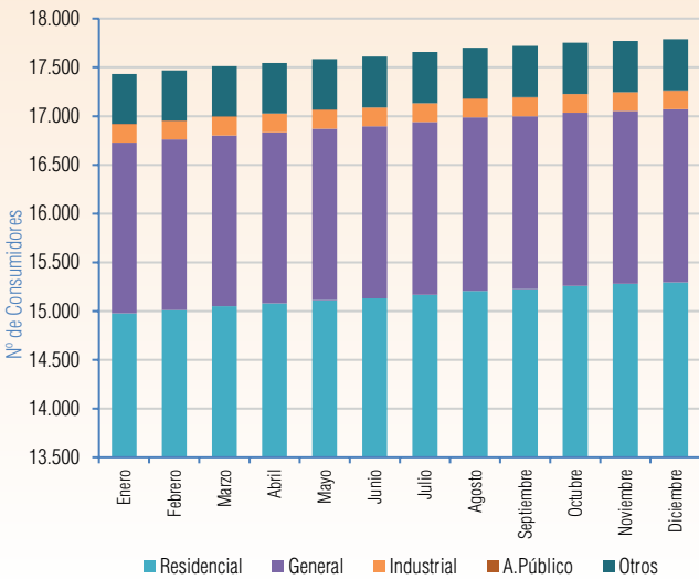
Gráfico V-44 Evolución mensual del número de Consumidores Gestión 2024 - CRE (Cordillera)
