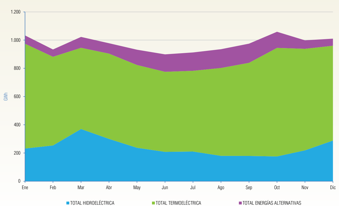
Gráfico II-10 Evolución mensual Centrales Hidroeléctrica, Termoeléctrica y E. Alternativa (GWh) Gestión 2024 - SIN
