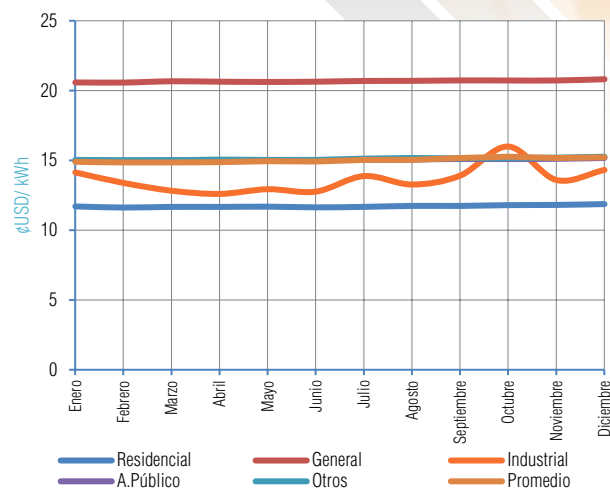
Gráfico V-286 Evolución Mensual de la Tarifa Promedio Gestión 2022 - ENDE (Cobija)
