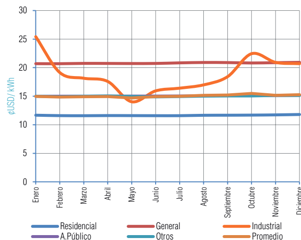
Gráfico V-292 Evolución Mensual de la Tarifa Promedio Gestión 2022 - ENDE (El Sena)
