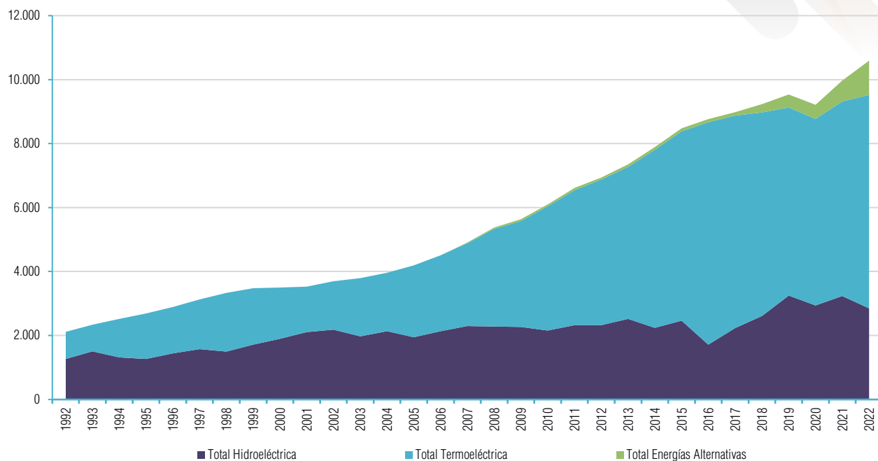
Gráfico II-15 Evolución Anual de la Generación Bruta Hidroeléctrica y Termoeléctrica (GWh) - SIN Período (1992 - 2022)
