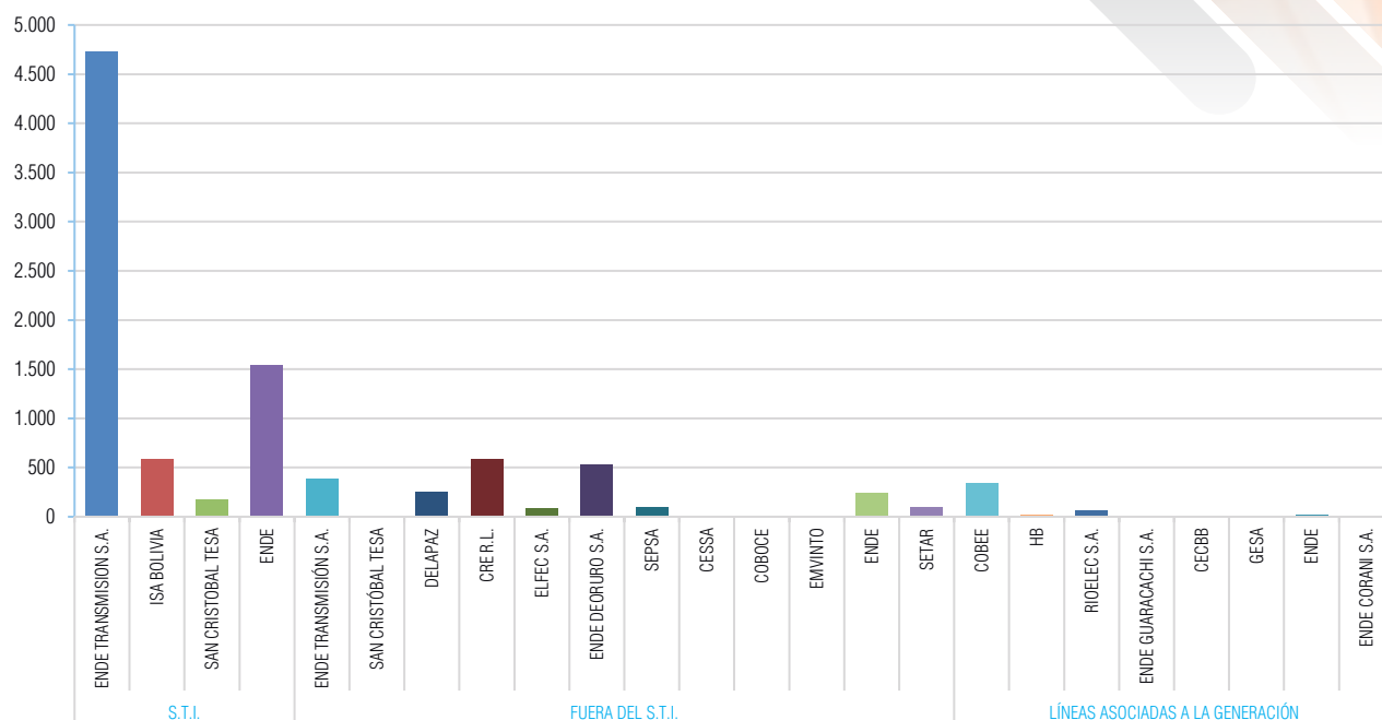
Gráfico II-6 Longitud de Línea de Transmisión (Km) Gestión 2022
