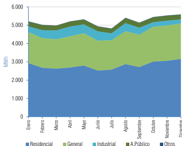
Gráfico V-284 Evolución mensual de ventas de Energía Gestión 2022 - ENDE (Cobija)
