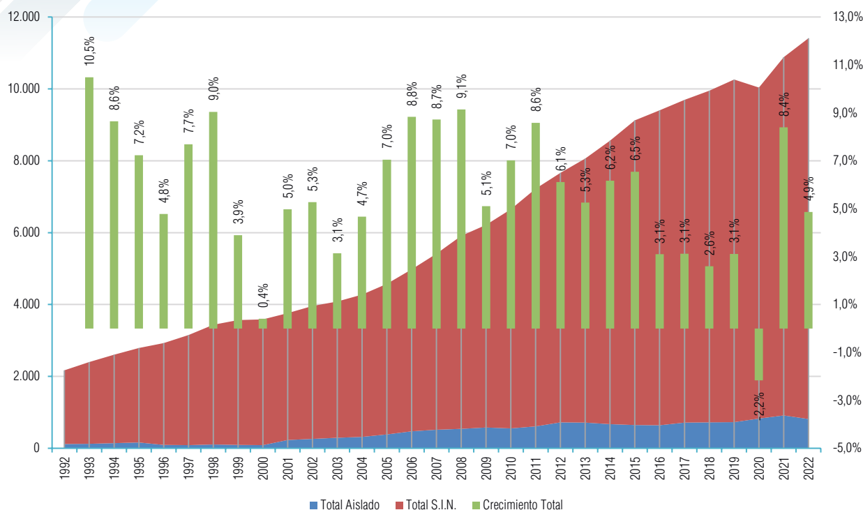
Gráfico I-9 Evolución anual de la Generación Bruta (GWh) - SIN y SA Periodo 1992 - 2022
