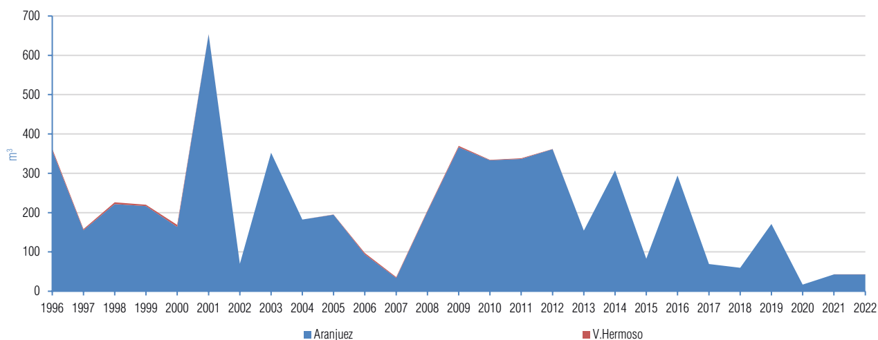
Gráfico IV - 7 Evolución anual del consumo de Diesel Oil en las centrales: Aranjuez y Valle Hermoso Período 1996 - 2022
