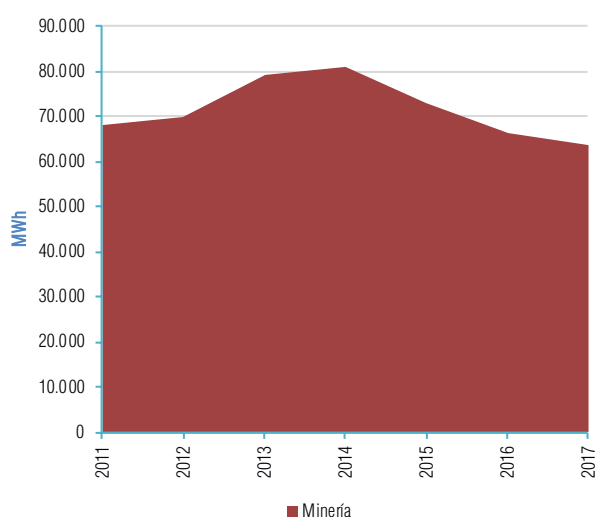
Gráfico V-93 Evolución de ventas de Energía Periodo (2011 - 2017) - SEPSA (San Bartolomé)
