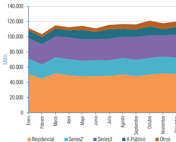
Gráfico V-52 Evolución mensual de ventas de Energía Gestión 2022 - ELFEC S.A.
