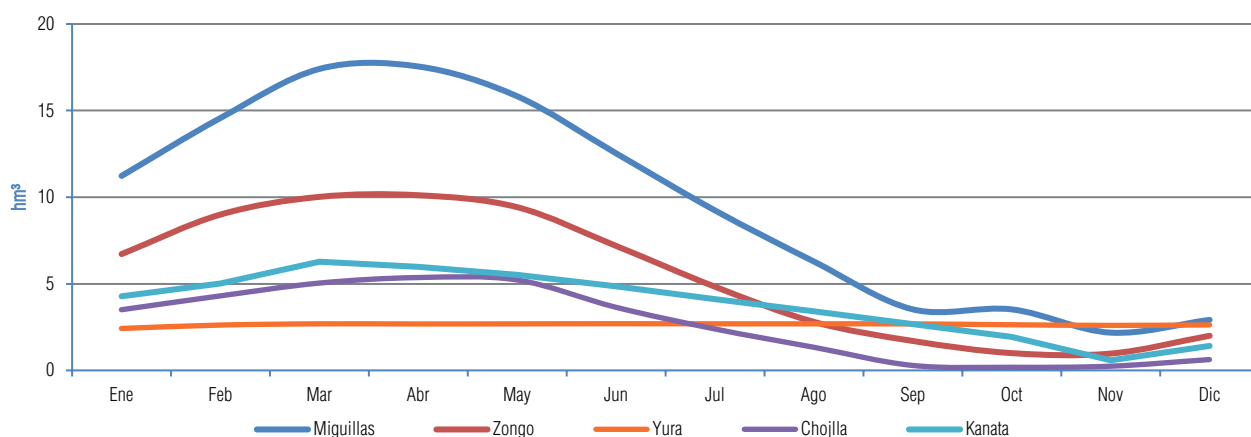
Gráfico IV - 15 Volúmen almacenado (hm 3 ) Miguillas, Zongo, Corani, Yura, Chojlla, Kanata Gestión 2022
