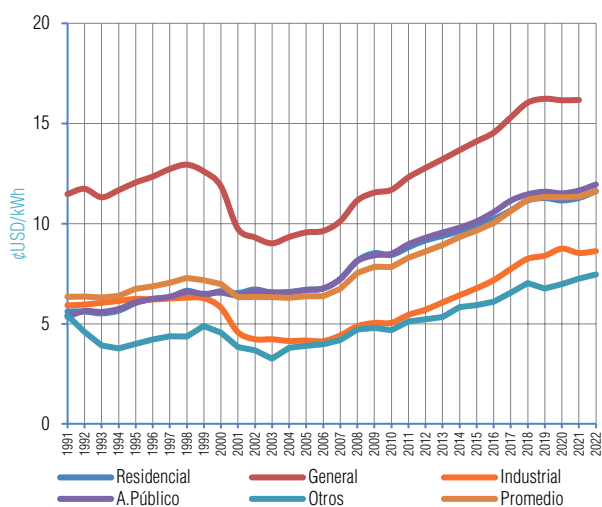
Gráfico V-53 Evolución de la Tarifa Promedio Periodo (1991 - 2022) - ELFEC S.A.
