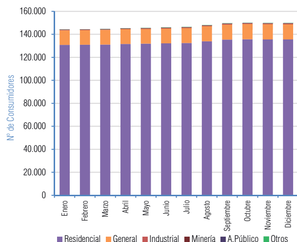
Gráfico V-62 Evolución mensual del número de Consumidores Gestión 2022 - ENDE DEORURO S.A.
