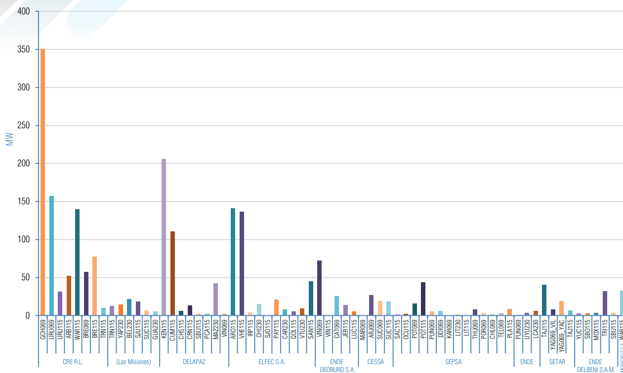
Gráfico II-17 Potencias máximas registradas en el nodo de retiro para Distribuidoras (MW) Gestión 2022 - MEM
