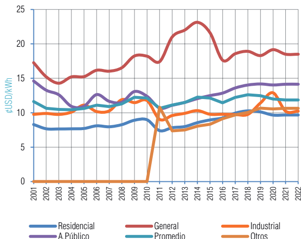
Gráfico V-216 Evolución de la Tarifa Promedio Periodo (2001 - 2022) - SETAR (Bermejo)
