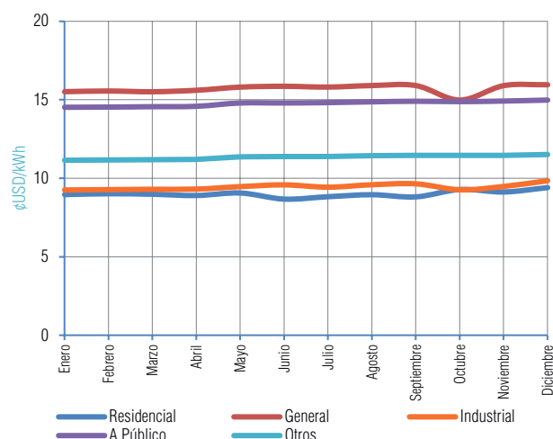
Gráfico V-120 Evolución Mensual de la Tarifa Promedio Gestión 2022 - ENDE DELBENI S.A.M. (San Borja)
