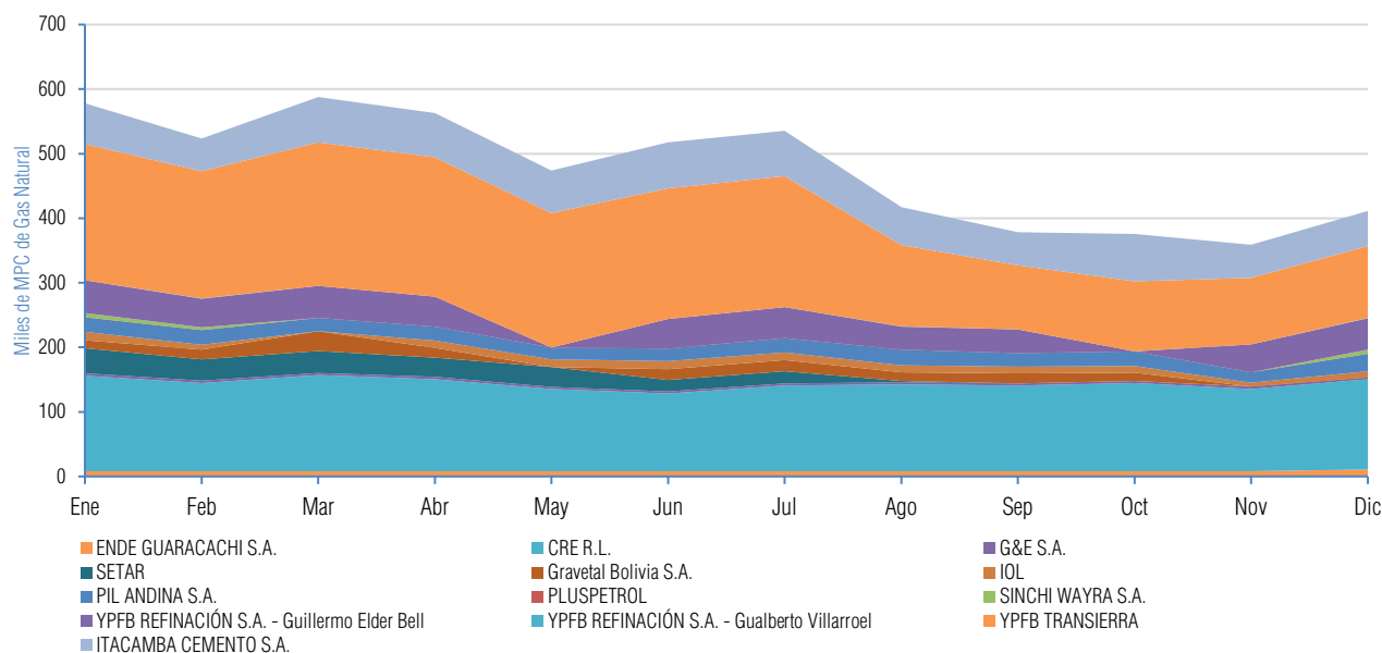
Gráfico VI-13 Evolución mensual consumo de Gas Natural (MMPC) Gestión 2022 - Sistemas Aislados
