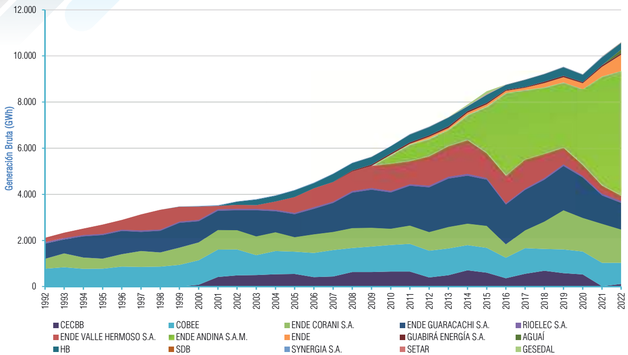
Gráfico II-13 Evolución anual Generación Bruta de las empresas (GWh) Período 1992-2022 - SIN
