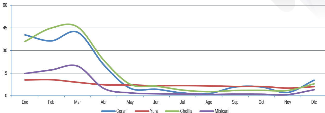
Gráfico IV - 12 Aportes a los embalses (hm 3 ) - Corani, Yura, Chojlla y Misicuni Gestión 2022
