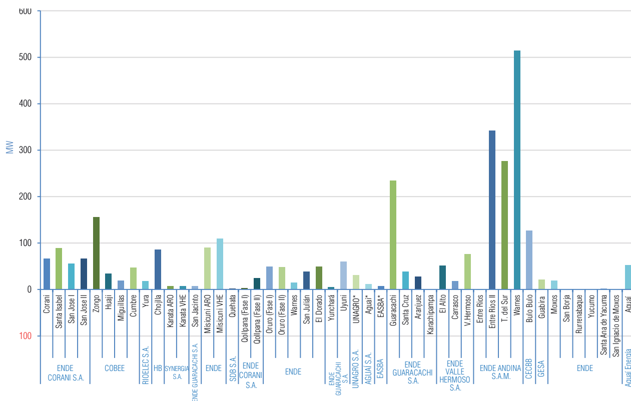
Gráfico II-18 Potencias máximas registradas en centrales de inyección Hidroeléctrica, Termoeléctrica y Energías Alternativas Gestión 2022 - MEM
