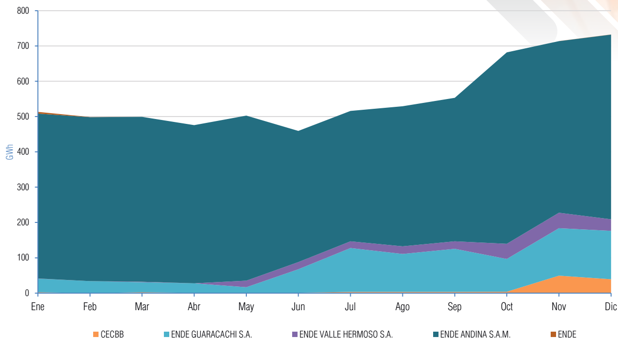
Gráfico II-12 Generación Termoeléctrica de las empresas (GWh) Gestión 2022 - SIN
