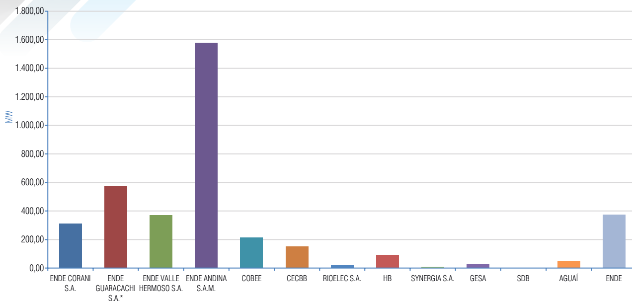
Gráfico II-2 Participación de las empresas del SIN Potencia Instalada (MW) Gestión 2022 - SIN
