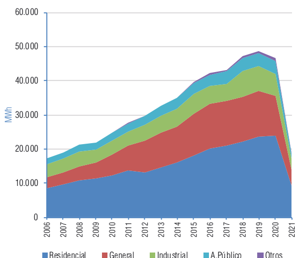
Gráfico V-277 Evolución de ventas de Energía Periodo (2006-2021) - CER (Riberalta)
