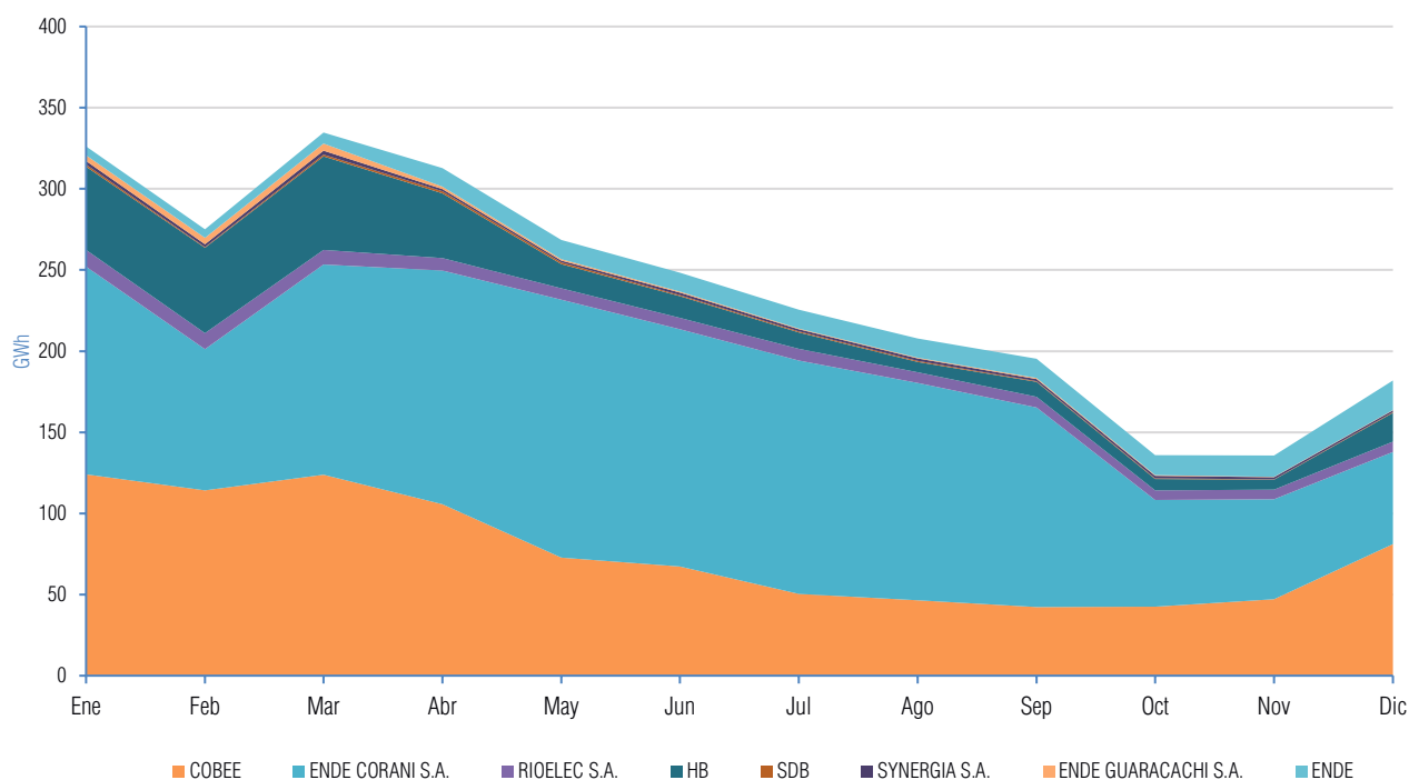
Gráfico II-11 Generación Hidroeléctrica de las empresas (GWh) Gestión 2022 - SIN
