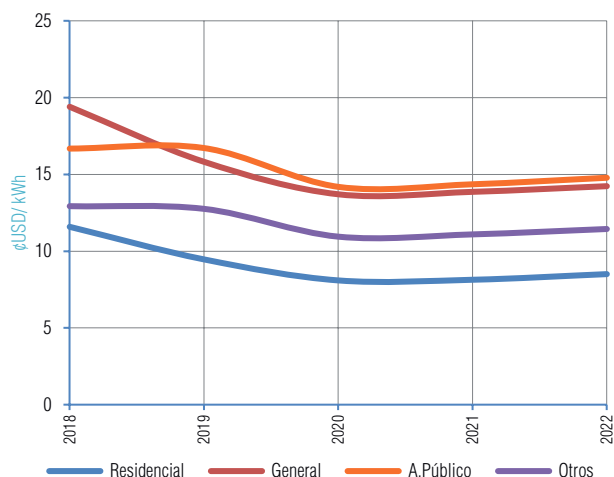
Gráfico V-327 Evolución de la Tarifa Promedio Periodo (2018 - 2022) - ENDE DELBENI S.A.M. (El Carmen de Iténez)
