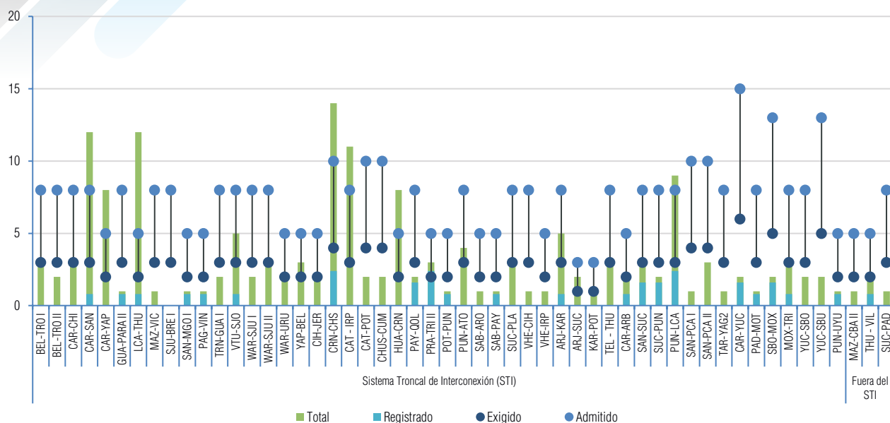
Gráfico VII-1 Número de desconexiones (veces) Periodo (Nov/2021 - Oct/2022) - Calidad de Transmisión
