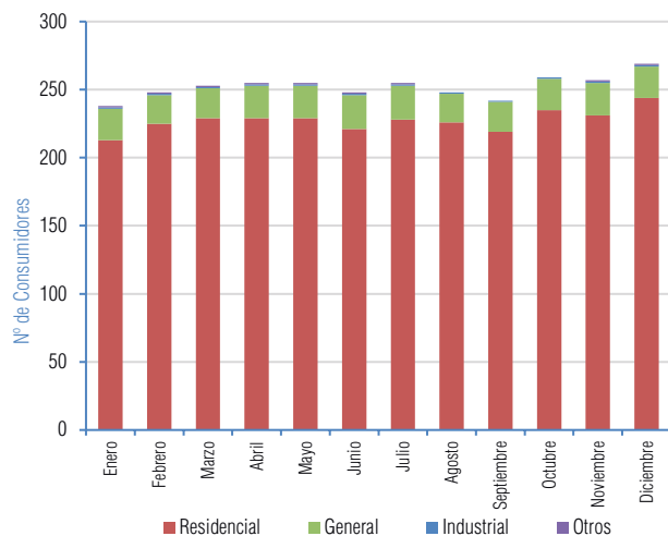
Gráfico V-306 Evolución mensual del número de Consumidores Gestión 2022 - ENDE (Villa Nueva)
