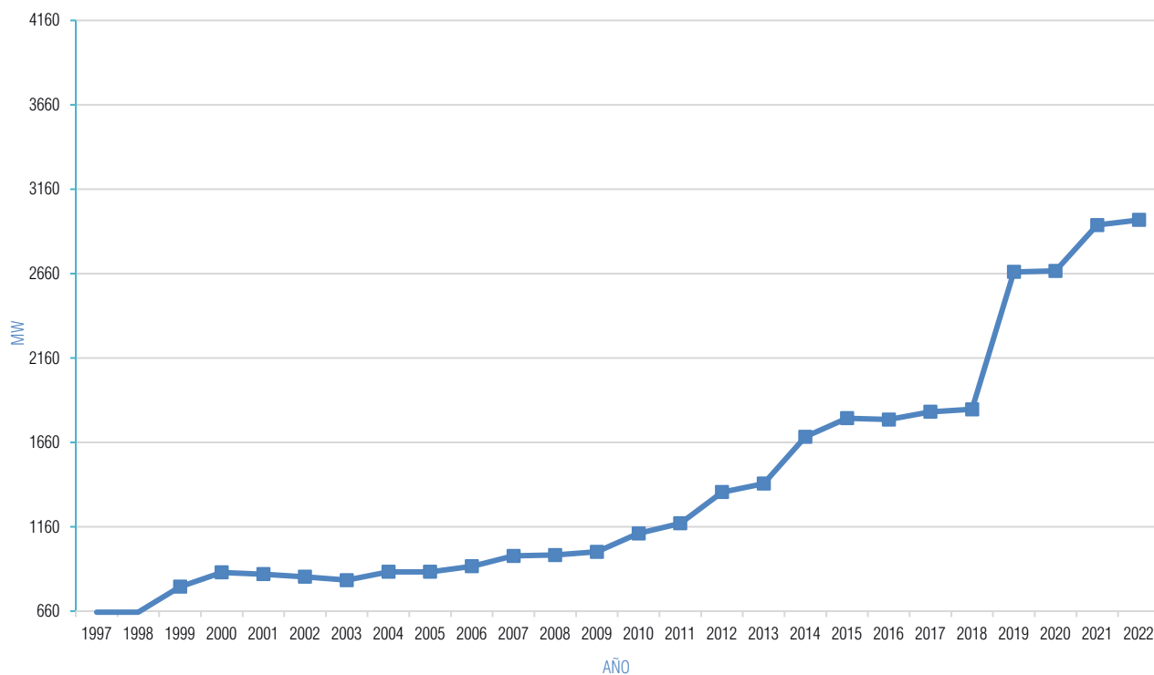
Gráfico I-5 Evolución de la Potencia Instalada Centrales Termoeléctricas SIN y SA (BOLIVIA) Periodo 1997-2022
