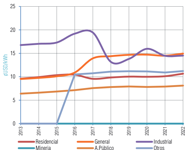
Gráfico V-155 Evolución de la Tarifa Promedio Periodo (2013 - 2022) - ENDE (Uyuni)
