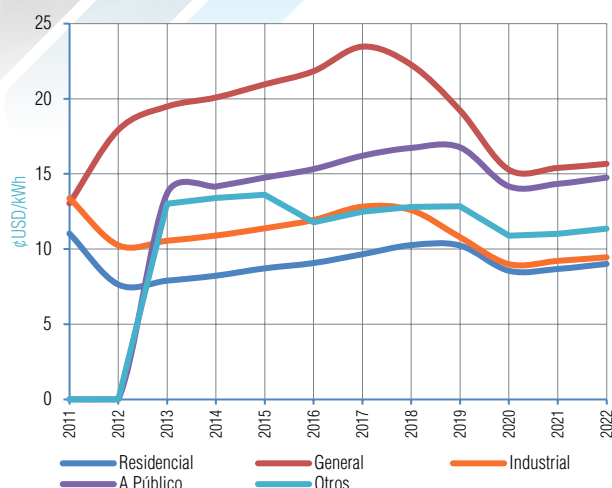
Gráfico V-119 Evolución de la Tarifa Promedio Periodo (2011 - 2022) - ENDE DELBENI S.A.M. (San Borja)
