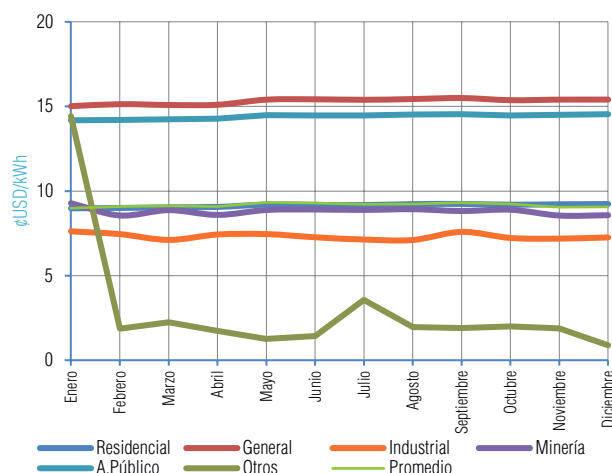
Gráfico V-72 Evolución Mensual de la Tarifa Promedio Gestión 2022 - SEPSA (Urbano)
