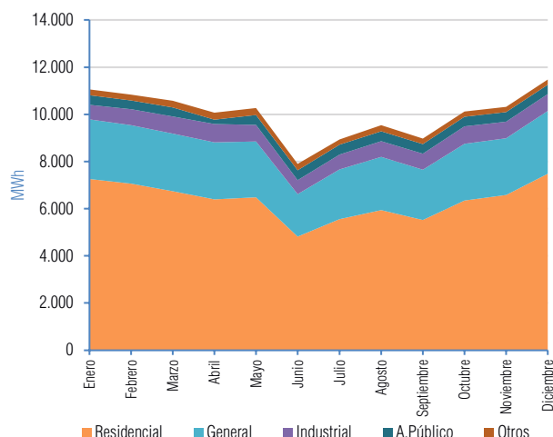
Gráfico V-100 Evolución mensual de ventas de Energía Gestión 2022 - ENDE DELBENI S.A.M. (Trinidad)
