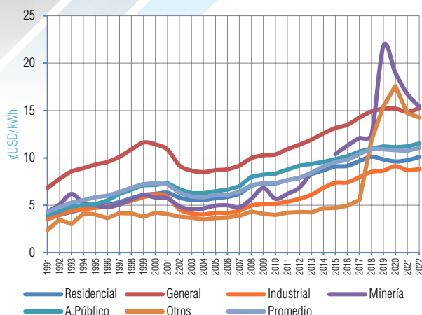
Gráfico V-17 Evolución de la Tarifa Promedio Periodo (1991 - 2022) - DELAPAZ
