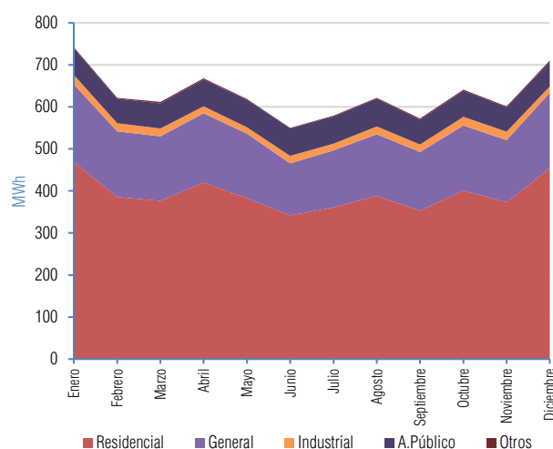
Gráfico V-124 Evolución mensual de ventas de Energía Gestión 2022 - ENDE DELBENI S.A.M. (Rurrenabaque)
