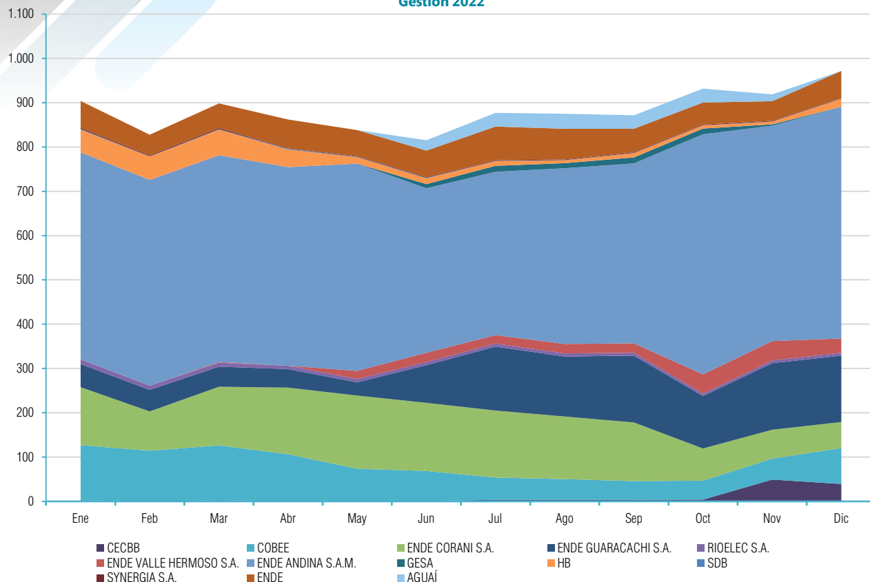
Gráfico I-8 Evolución mensual de la Generación Bruta en el SIN (GWh) Gestión 2022
