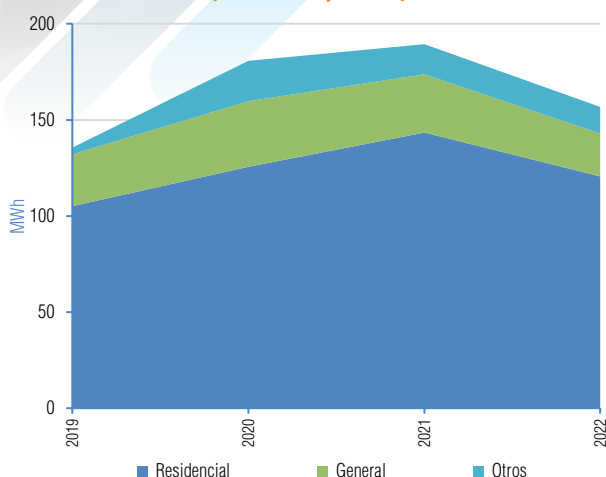
Gráfico V-343 Evolución de las ventas de Energía Periodo (2019 - 2022) - ENDE DELBENI S.A.M. (Cachuela Esperanza)
