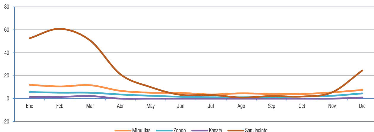
Gráfico IV-13 Aportes a los embalses (hm 3 ) - Miguillas, Zongo, Kanata y San Jacinto Gestión 2022
