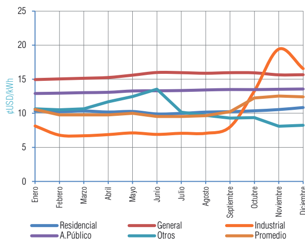
Gráfico V-241 Evolución mensual de la Tarifa Promedio Gestión 2022 - CRE R.L. (G. Busch)
