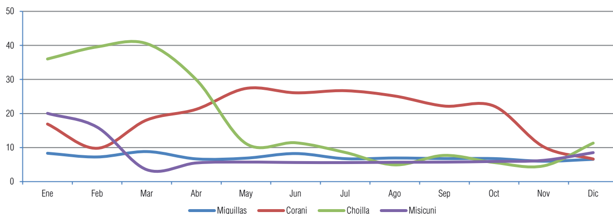
Gráfico IV - 10 Volúmen utilizado de los embalses (hm³) - Miguillas, Corani, Chojlla y Misicuni Gestión 2022
