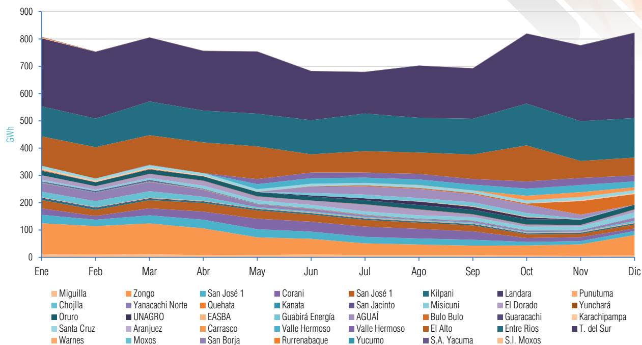
Gráfico II-9 Evolución mensual Generación Bruta de Centrales (GWh) Gestión 2022 - SIN
