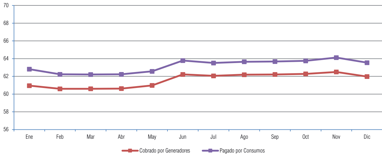
Gráfico III-8 Precio Potencia Firme y Punta (Bs/MW) Gestión 2022 - MEM
