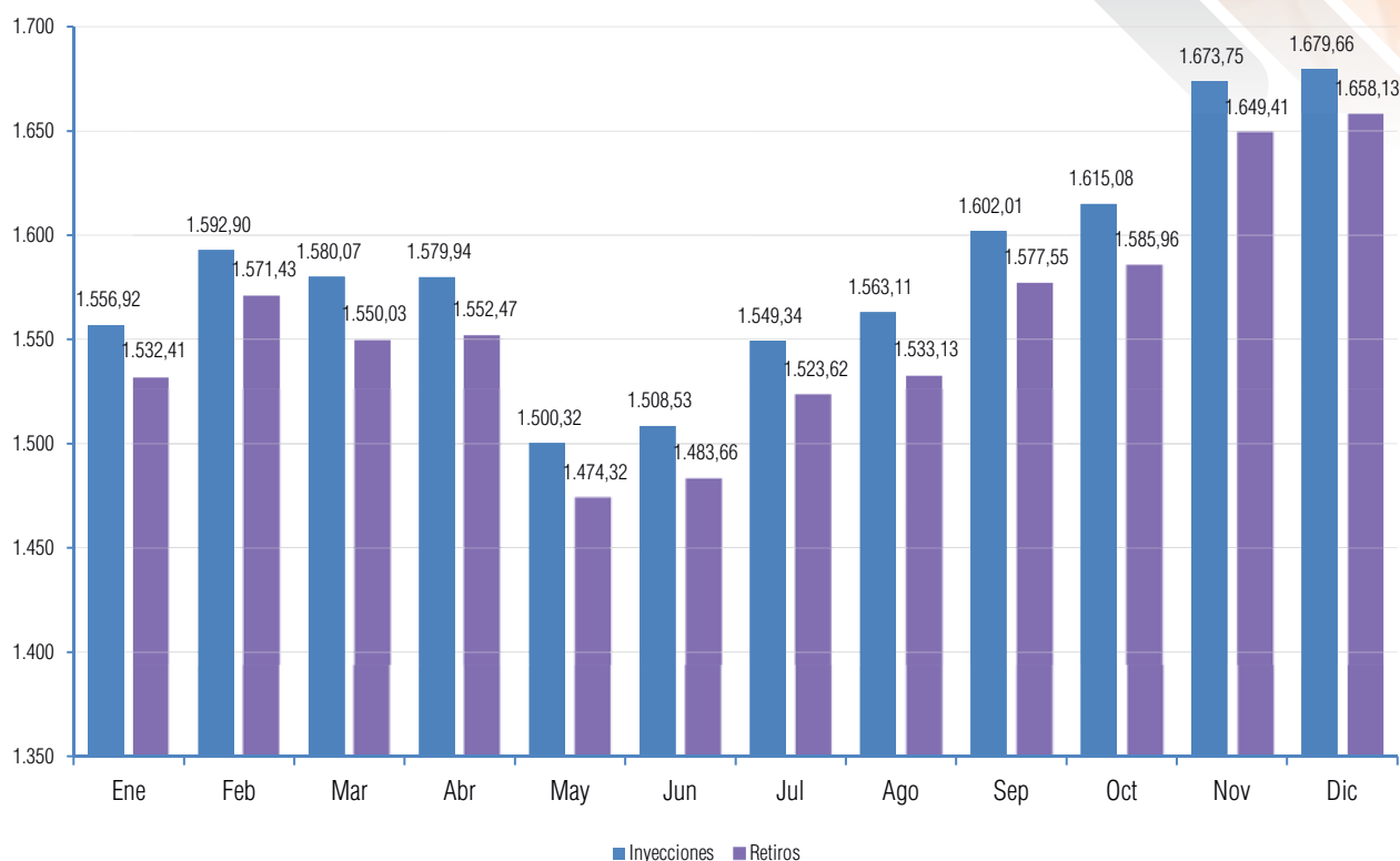
Gráfico II-19 Potencia Máxima (MW) Gestión 2022 - MEM
