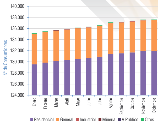
Gráfico V-32 Evolución mensual del número de Consumidores Gestión 2022 - DELAPAZ (Sistema Nuevo)
