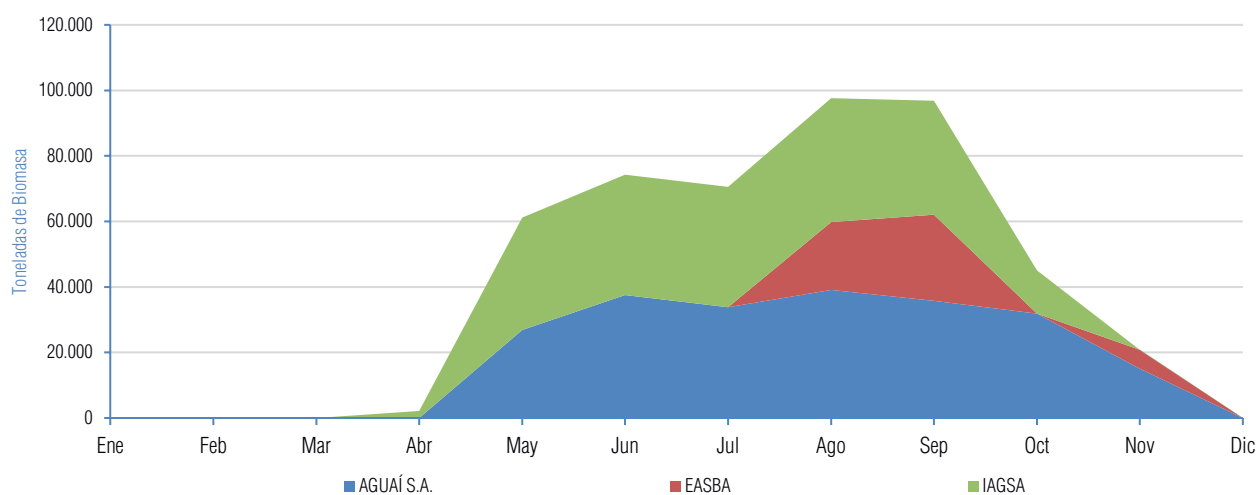
Gráfico VI-15 Evolución mensual del consumo de Biomasa (Tn) Gestión 2022 - AGUAÍ S.A., EASBA e IAGSA
