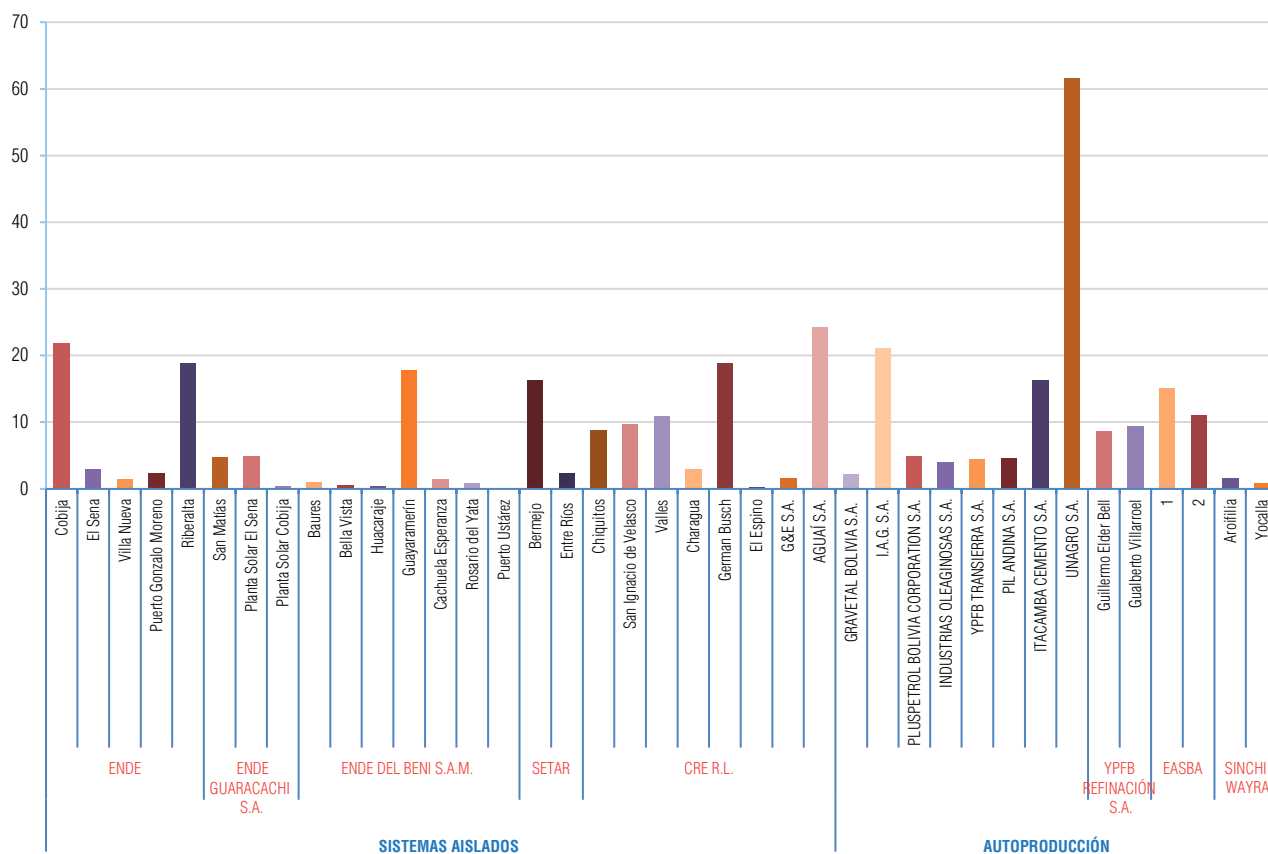
Gráfico VI-7 Potencia Efectiva S.A. y Autoprodutores (MW) Gestión 2022
