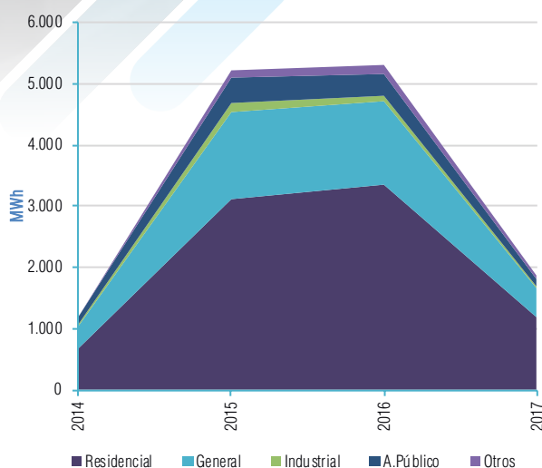
Gráfico V-141 Evolución anual de ventas de Energía Periodo (2014 - 2017) - ENDE DELBENI S.A.M. (Yacuma)
