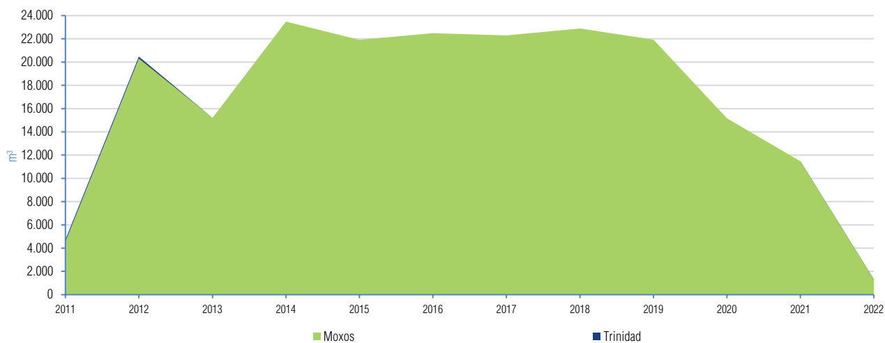
Gráfico IV - 8 Evolución anual del consumo de Diesel Oil en las centrales: Moxos y Trinidad Período 2011 - 2022
