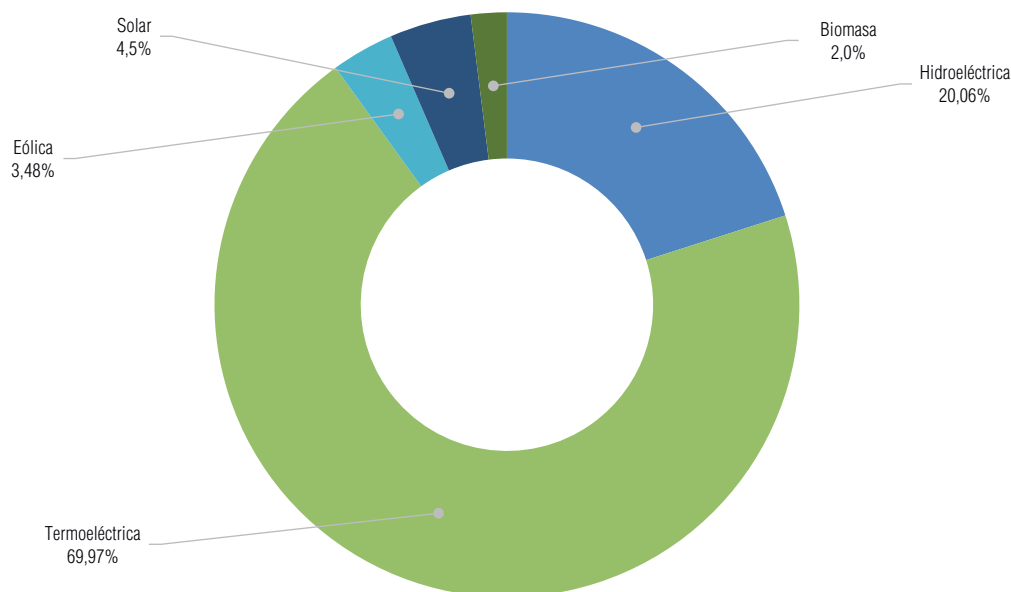
Gráfico II-1 Potencia Instalada en el SIN por tipo de tecnología Gestión 2022
