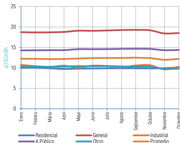
Gráfico V-180 Evolución mensual de la Tarifa Promedio Gestión 2022 - SETAR (Yacuiba)
