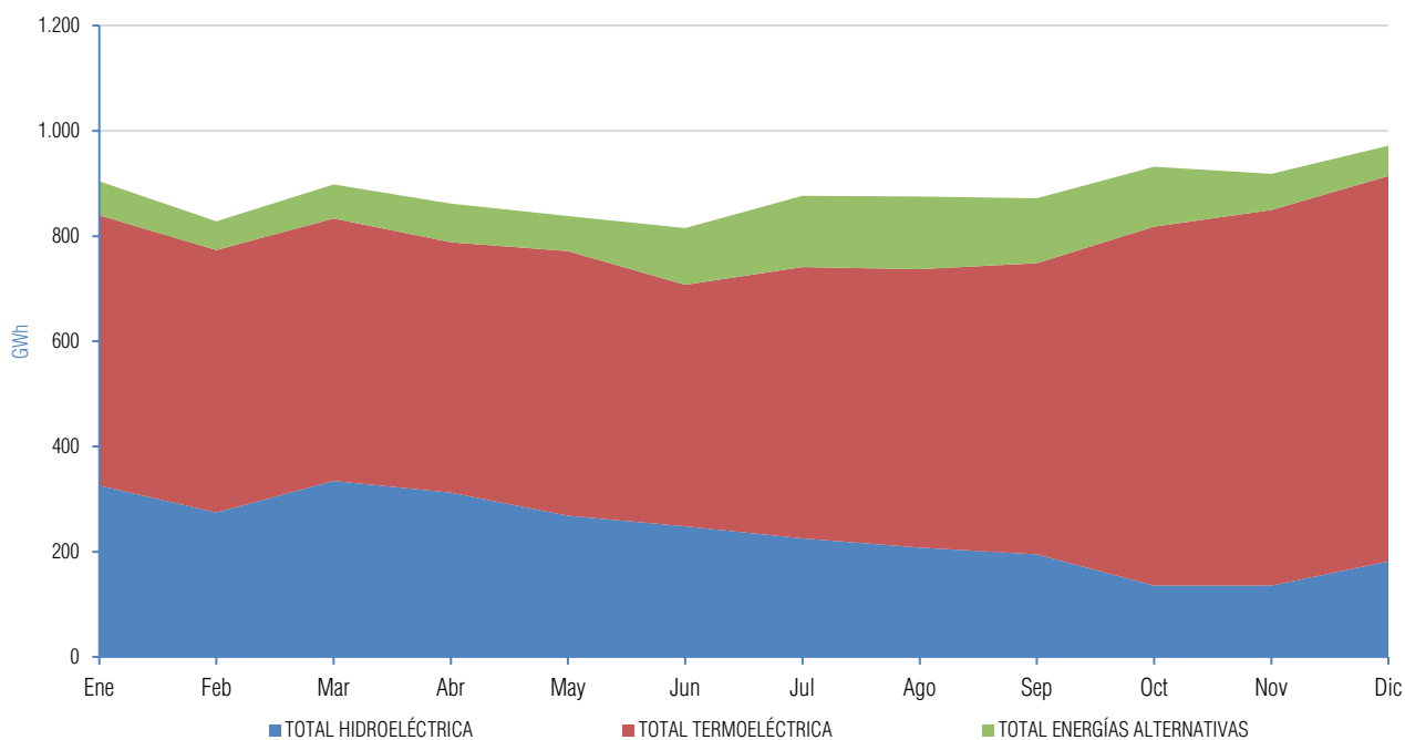
Gráfico II-10 Evolución mensual Centrales Hidroeléctricas, Termoeléctricas y E. Alternativas (GWh) Gestión 2022 - SIN
