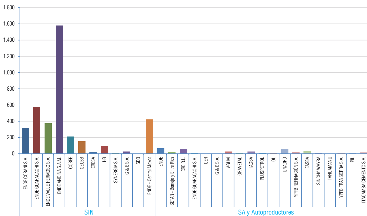
Gráfico I-3 Potencia Instalada por empresa (MW) Gestión 2022 - SIN y SA
