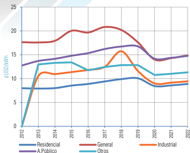
Gráfico V-131 Evolución de la Tarifa Promedio Periodo (2012 - 2022) - ENDE DELBENI S.A.M. (Santa Rosa)
