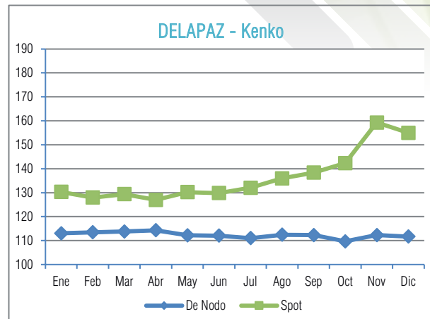
Gráfico III-6 Precios de nodo Vs. Precios Spot de la energía (Bs/MWh con IVA) Gestión 2022 - MEM
