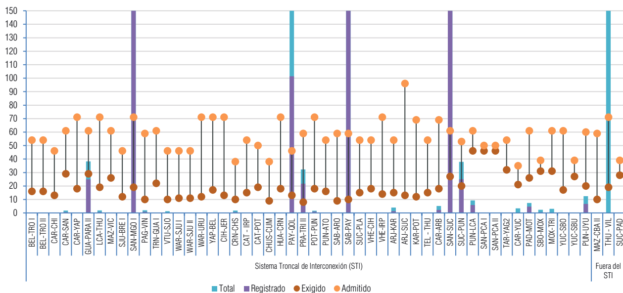
Gráfico VII-2 Duración media de desconexiones (minutos) Periodo (Nov/2021-Oct/2022) - Calidad de Transmisión
