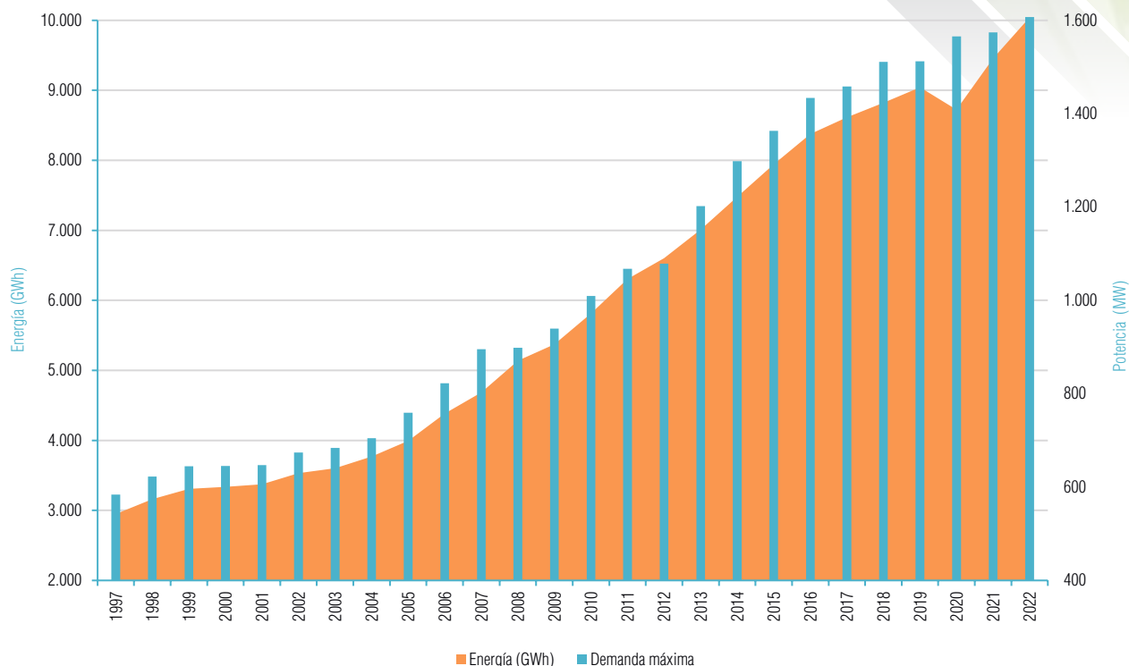
Gráfico III-5 Evolución anual de la demanda de Electricidad Periodo (1997-2022) - MEM
