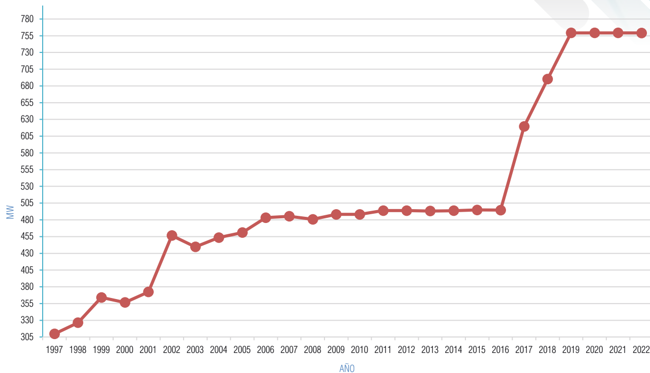
Gráfico I-4 Evolución de la Potencia Instalada Centrales Hidroeléctricas SIN y SA (BOLIVIA) Periodo 1997-2022
