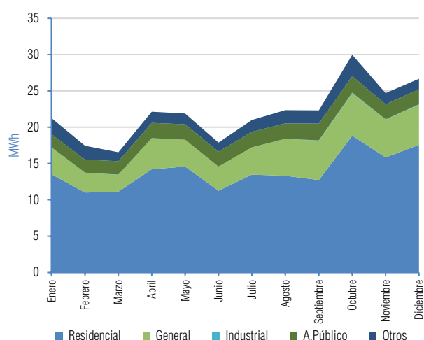
Gráfico V-332 Evolución de las ventas de Energía Gestión 2022 - ENDE DELBENI S.A.M. (Exaltación)
