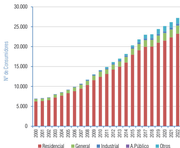
Gráfico V-230 Evolución número de Consumidores Periodo (2000 - 2022) - CRE R.L. (Valles Cruceños)
