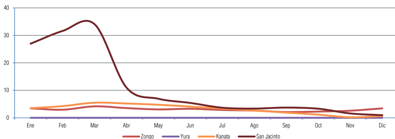
Gráfico IV - 11 Volúmen utilizado de los embalses (hm³) - Zongo, Yura, Kanata y San Jacinto Gestión 2022
