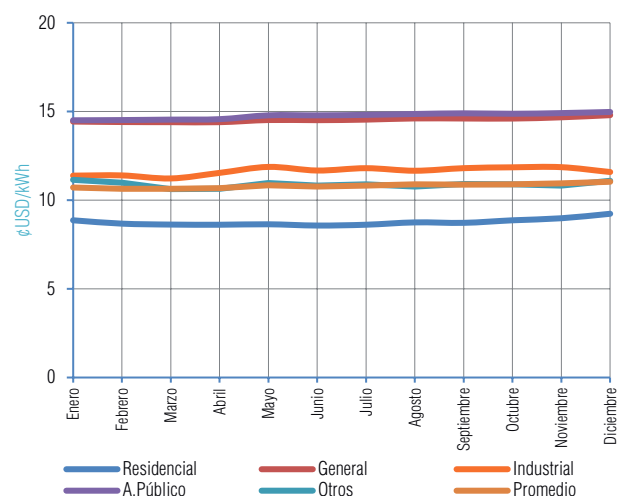
Gráfico V-138 Evolución mensual de la Tarifa Promedio Gestión 2022 - ENDE DELBENI S.A.M. (Reyes)
