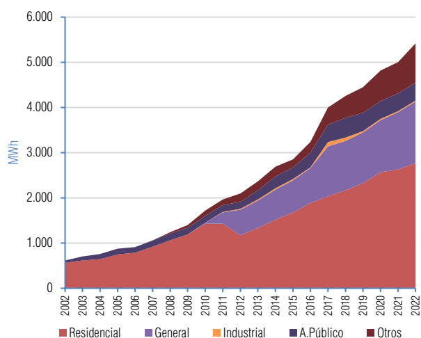
Gráfico V-244 Evolución de Ventas de Energía Periodo (2002- 2022) - CRE R.L. (Charagua)
