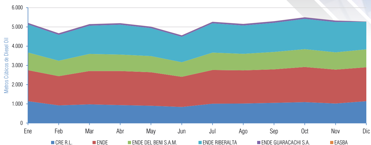
Gráfico VI-14 Evolución mensual consumo de Diesel Oil (m³) Gestión 2022 - Sistemas Aislados
