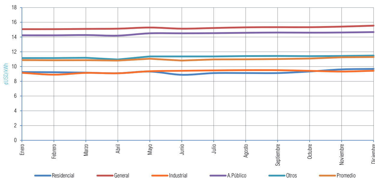
Gráfico V-407 Evolución mensual de la Tarifa Promedio Gestión 2022 - ENDE DELBENI S.A.M.
